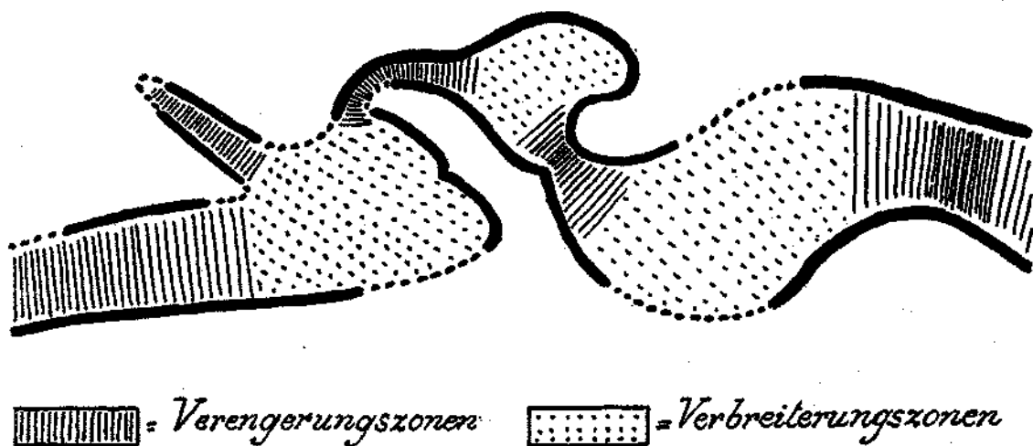
Fig. 1. Umformung des Innenfeldes der mediterranen Faltenzonen.
