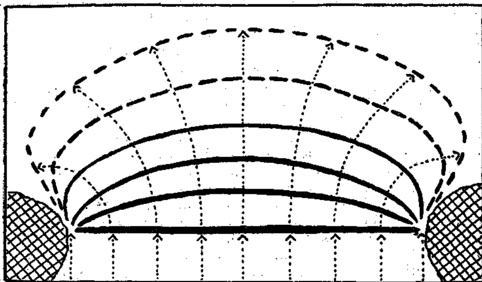
Fig. 4. Schema des Vorlaufbogens in verschiedenen Stadien. Ergebnis der Streckung = Verdoppelung der Ausgangslänge.
