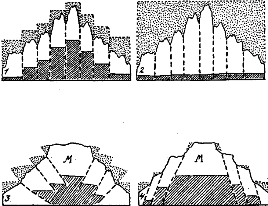
Fig. 15. Schraffiert = unterer, Weiß = oberer Teil einer Schichtfolge. Punktiert = die von der Erosion bereits entfernten Massen. 1 = Zerlegung mit vertikalen Schubflächen. Vertikalverschiebungen. 2 = Zerlegung mit vertikalen Schubflächen. Horizontalverschiebungen. 3 = Zerlegung mit konvergierenden Schubflächen. 4 = Zerlegung mit divergierenden Schubflächen. M = Ausbildung eines bevorzugten Mittelteiles.
