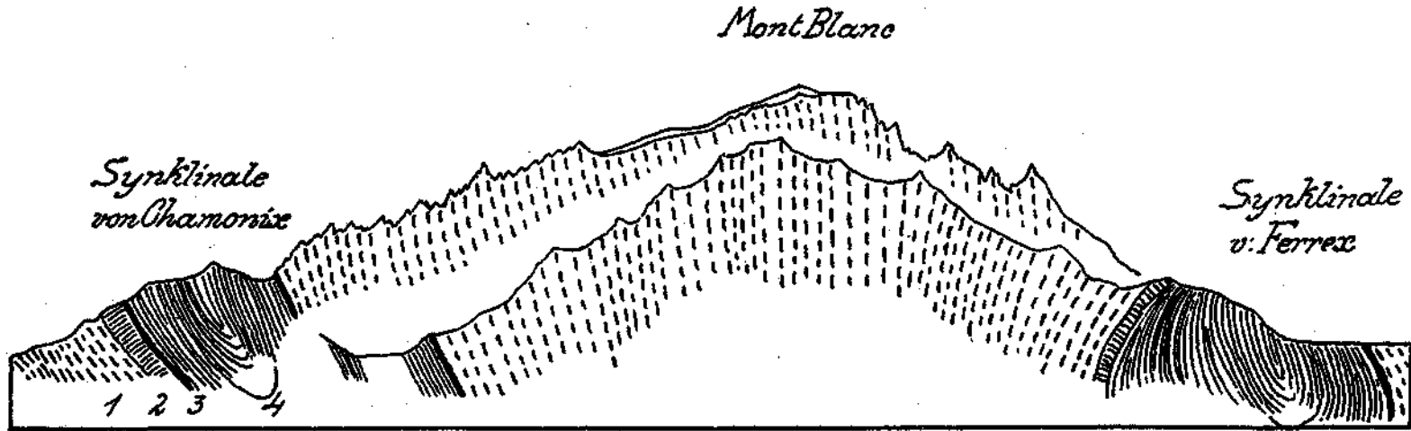
Fig. 17. Schematische Kopie des Montblanc-Profiles in der Geologie der Schweiz von A. Heim. 1 = Granit und kristalline Schiefer, 2 = Carbon, 3 = Trias, 4 = Jura.
