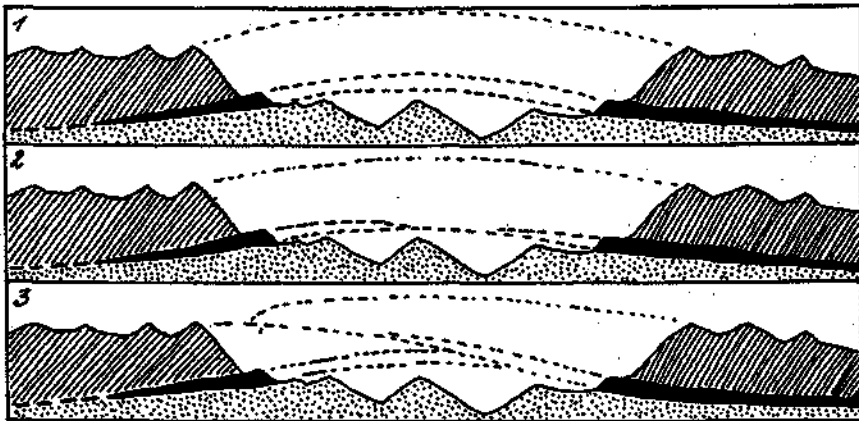
Fig. 8. Punktiert = tektonisch einheitliches Grundgebirge. Schwarz und schraffiert = Schubmassen die darauf lagern. 1 = Kombination zu zwei je zusammenhängenden Schubdecken. 2 = Kombination von zwei getrennten liegenden, mit einer hangenden Schubdecke. 3 = Kombination von je zwei sich übergreifenden Schubdecken.
