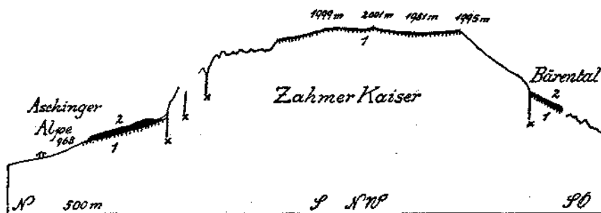
Fig. 16. 1 = Reste einer alten EinrundungsOberfläche. 2 = Gehängebreccien. x = junge Schubflächen, an denen die Heraushebung des Gipfelkörpers vollzogen wurde.
