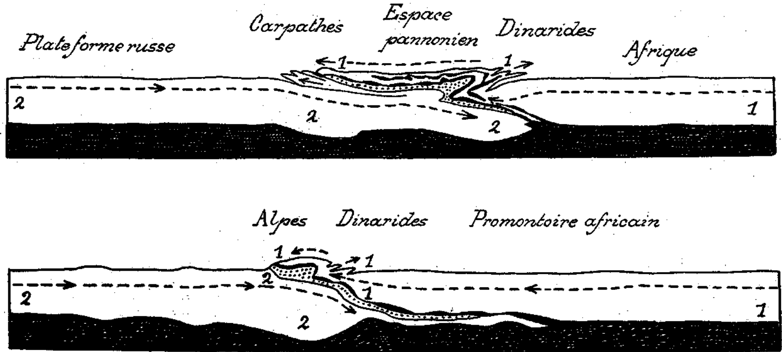
Fig. 3. 1 = Africa-Gondwana-Masse, 2 = Eurasien.
