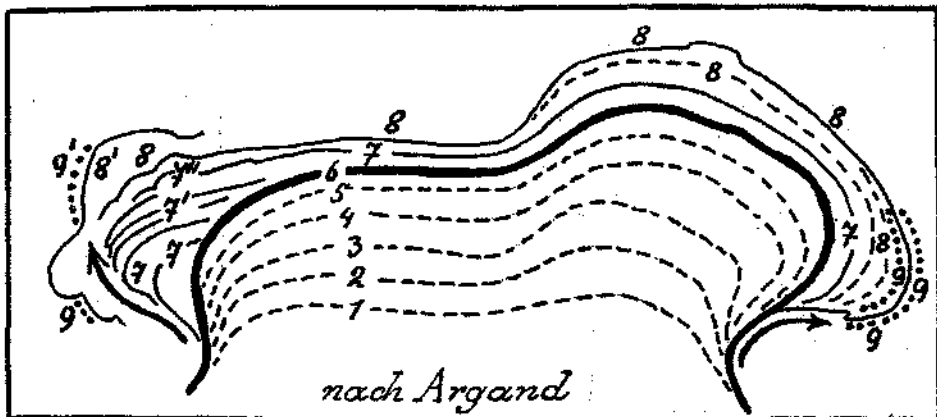
Fig. 2. Progression des fronts alpino-carpathiques. ca. 1:17,000,000 1 à 9, progression des fronts du Jurassique au Quaternaire. 1 à 6, progression au Jurassique et à l'Éocretacé. 6, front des nappes au moment du premier paroxysme. 7 à 9, nappes à paroxysme tertiaire. 7, 7', 7'', progressions au Nummulitique. 8, au Néogène. 9, au Néogène supérieur et au Quaternaire. Les flèches indiquent le sens des dérives. 8', 9', progressions frontales du Jura. 8', au Néogène moyen. 9', au Néogène supérieur et au Quaternaire.
