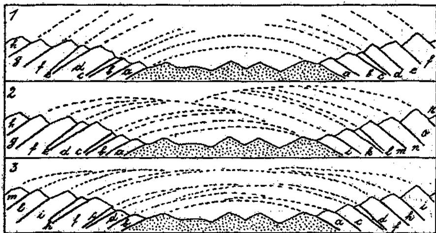
Fig. 9. Punktirt = tektonisch einheitliches Grundgebirge. a - r = einzelne Schubdecken. 1 = Kombination mit paarweiser Gleichstellung. 2 = Kombination als 2 getrennte sich übergreifende Deckensysteme. 3 = Kombination mit mehrfach abwechselndem Übergreifen.
