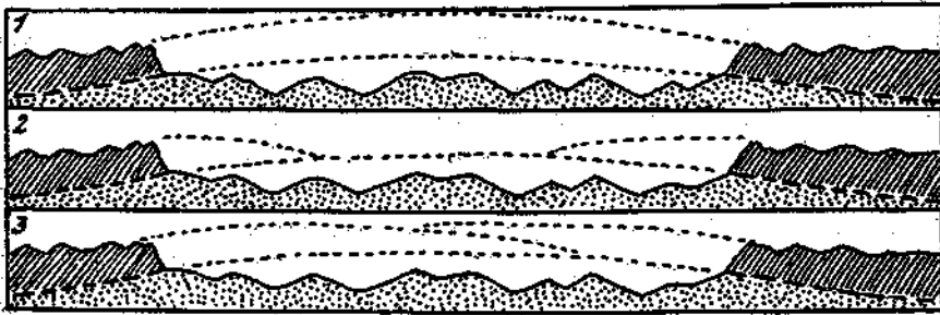
Fig. 7. Punktiert = tektonisch einheitliches Grundgebirge. Schraffiert = darauf liegende Schubmassen. 1 = Kombination zu einer Schubdecke. 2 = Kombination zu zwei ganz getrennten Schubdecken. 3 = Kombination zu zwei einander übergreifenden Schubdecken.
