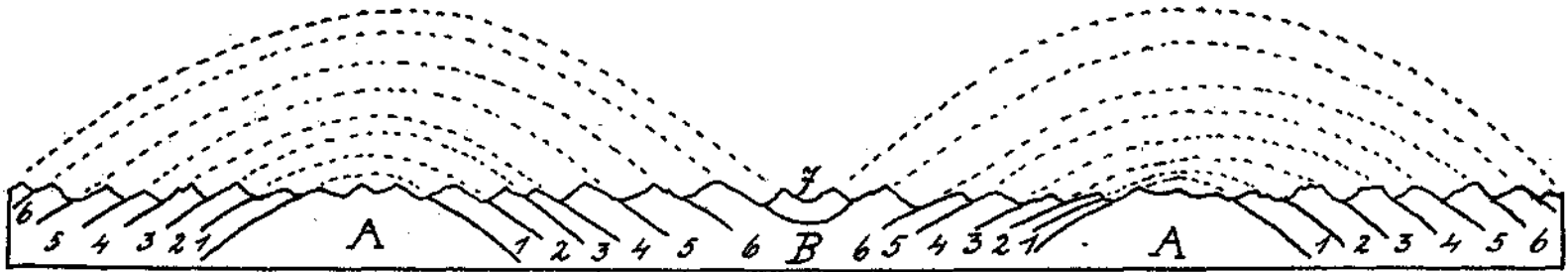
Fig. 10. A = Kulmination, B = Depression von Decken. Diese Art von Zählung und Parallelisierung der Decken ergibt ein Maximum für die theoretisch nötige Höhe der Kulminationen und erfordert eine riesige Abtragung.
