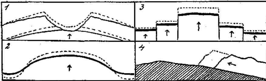
Fig. 13. Beispiele von Jungtektonik im Sinne des alten Baustils. 1 = Weiterbiegung eines zerschnittenen Gewölbes. 2 = Verstärkung der Herauswölbung. 3 = Verstärkung der Staffelung. 4 = Weiterschub einer Schubmasse.
