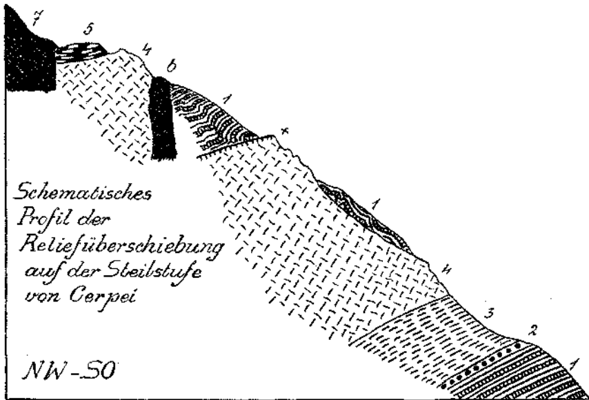
Fig. 8. 1 = Werfener Schichten. 2 = Richtofonkonglomerat. 3 = Unterer Muschelkalk. 4 = Mendoladolomit. 5 = Buchensteiner Schichten. 6 = Porphyritgang. 7 = Tuffe und Laven. x = Schöne Schubbfläche.
