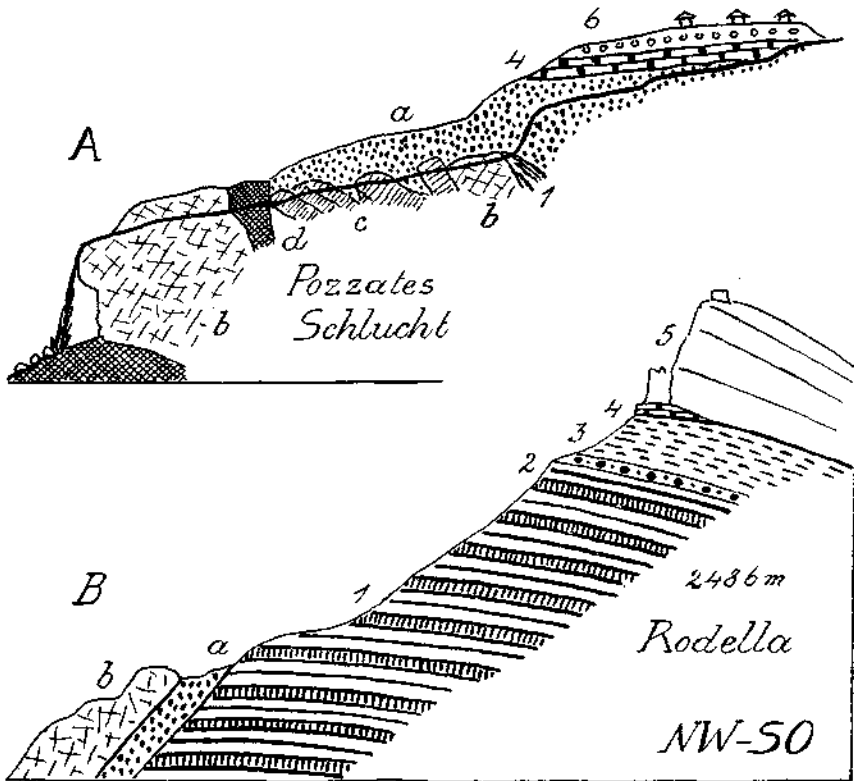
Fig. 7. 1 = Werfener Schichten. 2 = Richthofenkonglomerat. 3 = Unterer Muschelkalk. 4 = Buchensteiner Schichten. 5 = Marmolatakalk. 6 = Tuffbreccien. a = Gehängeschuttbreccie. b = Mendoladolomit. c = Geschichtete, feingebänderte Dolomite. d = Porphyritgänge.
