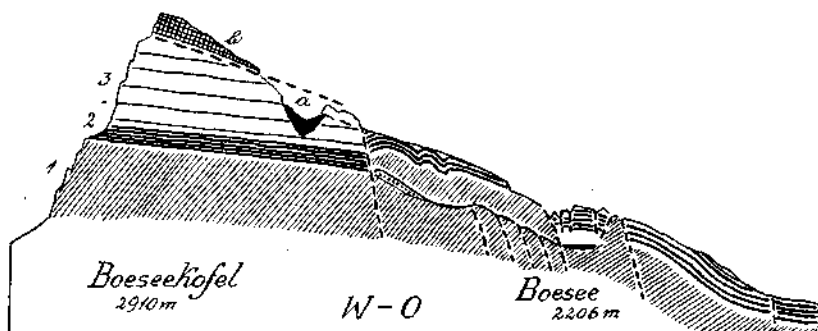
Fig. 6. 1 = Schlerndolomit. 2 = Raibler Schichten. 3 = Dachsteindolomit. a = Füllmasse, zumeist aus Neokom. b = Schubshölle aus Dachsteindolomit.
