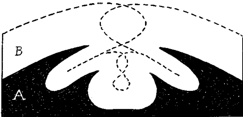
Fig. 2. Das Schema stellt einen schwarzgezeichneten Faltenunterbau — A — dar. Der Oberbau — B — kann trotz starker Ausquetschungen der Vorzeichnung des Unterbaues nicht mehr folgen. Seine Faltungen würden sich dabei bereits gegenseitig übergreifen und sind daher nicht ausführbar.
