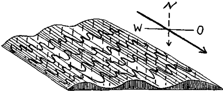
Fig. 2. Der starke Pfeil zeigt die Richtung der großen Eisschliffrienen an, die unterbrochenen Linien deuten ein jüngeres Ritzensystem an. Schichtstreichen = O—W mit intensiver Fältelung.
