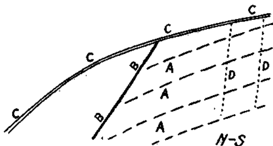
Fig. 9. Verteilung der Bewegungsbahnen im Körper der Sulzfluh.
