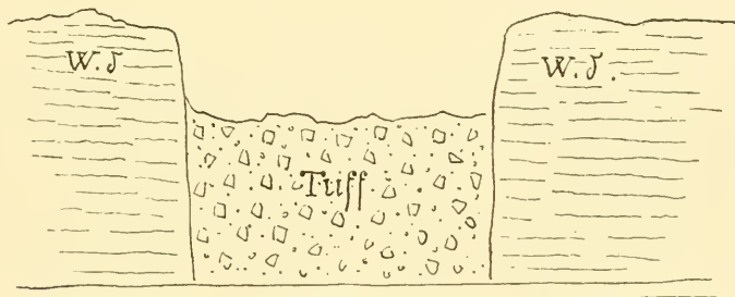
Fußweg Gang im Mohrenteich-Thale Fig. 36.
