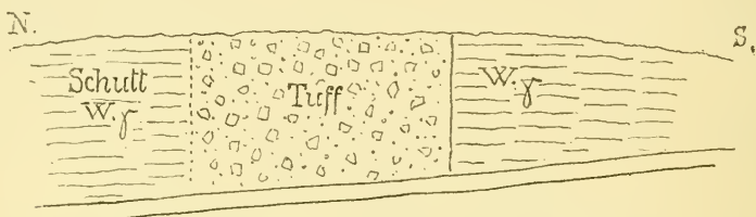
Steige v. Neuffen nach Hülben. Unterer Gang. Fig. 23.
