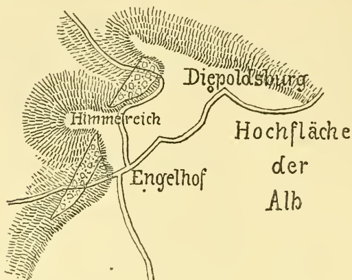
Gang beim Engelhof, vergr. Bild d. geol. K. v. W. Fig. 12.
