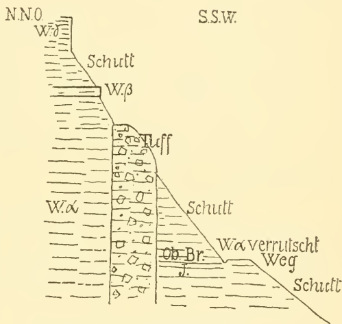
Tuffgang im buckelten Teich Fig. 33.
