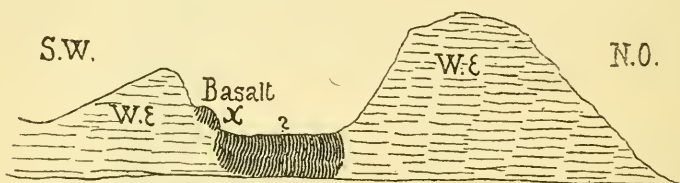
Basalt-Maardes Dintebühl, Profil von A nach B der Fig. 104.
