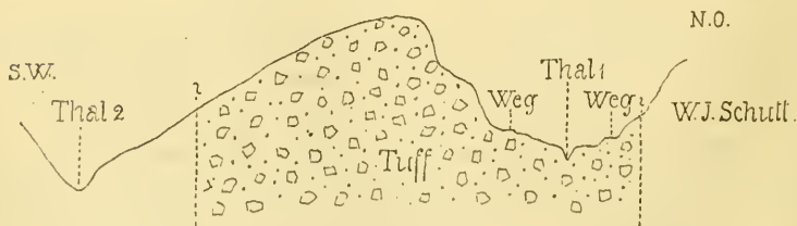
2 tes Profil im südlichen Teil des Maars v. Hengen Fig. 3.
