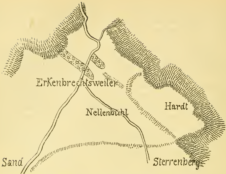
Die beiden Gänge bei Erkensbrechtsweiler Vergröfs. Kartenbild. d. geolog. K. v. Württemberg Fig. 5.
