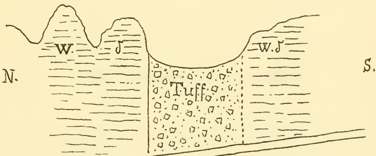
Gang im Riedheimer Thal Fig. 39.
