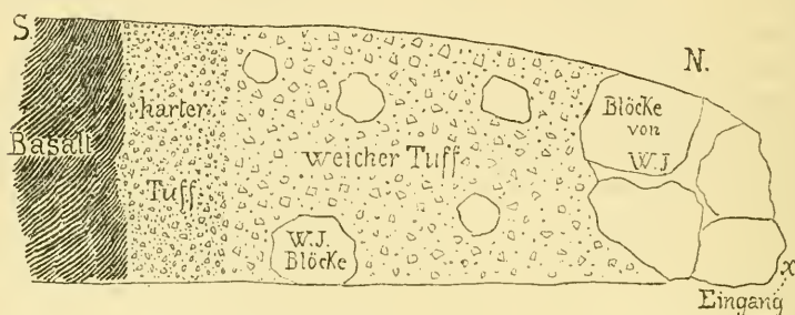
Gözenbrühl Profil des durch den Tuff in den Basaltkern getriebenen Weges Fig. 62
