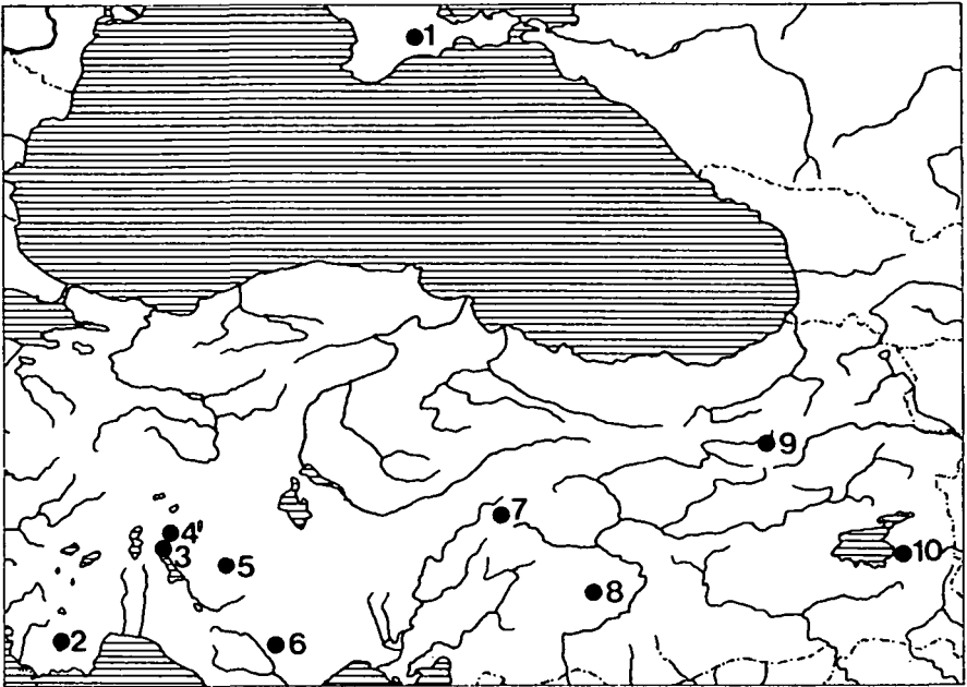
Karte 1. Verbreitung von Rophites clypealis .
