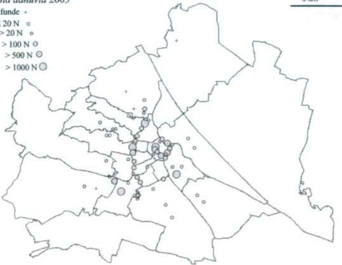
Abb. 2: Nestaggregationen von Andrena danuvia 2003 in Wien (Bezirks- und Landesgrenzen). Sie sind nach ihrer Größe (Anzahl N gezählter Nesteingänge) in fünf Kategorien unterteilt. Bei den mit + gekennzeichneten Einzelfunden lebender oder toter Tiere konnten keine Nesteingänge am Standort gefunden werden. Zu jedem Fundpunkt findet sich ein entsprechender Eintrag in Tab. A.
