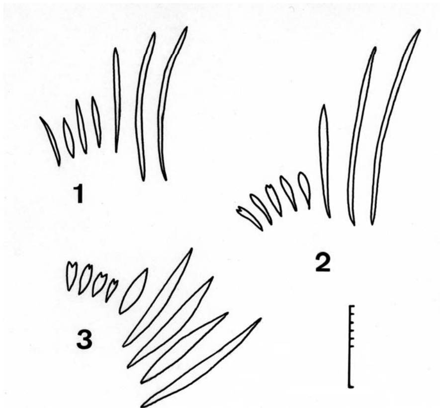
Abb. 1-3: Schuppen am Vorderflügel zwischen Diskoidalzelle und Außenrand bei Montanima karavankensis ( Abb. 1 ; Petzen), M. venetiana ( Abb. 2 ; Foppolo) und M. predotae ( Abb. 3 ; Lectotypus). Jeweils links die Grundschruppen, rechts die Deckschruppen. Maßbalken gesamt 0.1mm.
