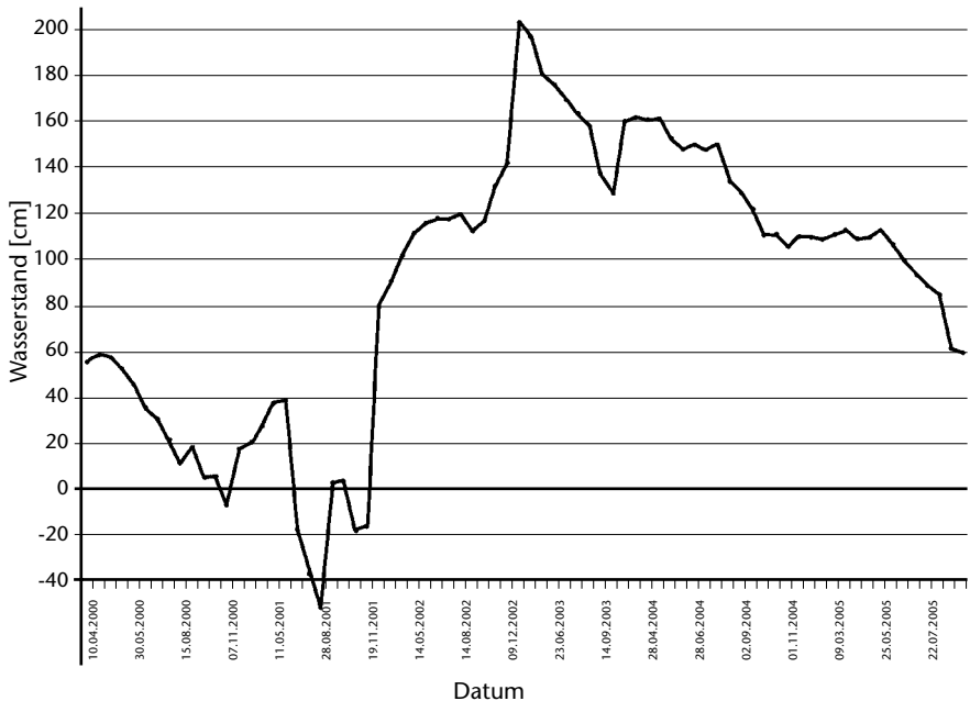
Abbildung 1: Wasserstandsverlauf im Zentrum des ÖÜB-Feldsolls bei Brodowin in den Jahren 2000 bis 2005. — Figure 1: Course of the water table at the kettle hole near Brodowin, Brandenburg, Germany from 2000 to 2005.
