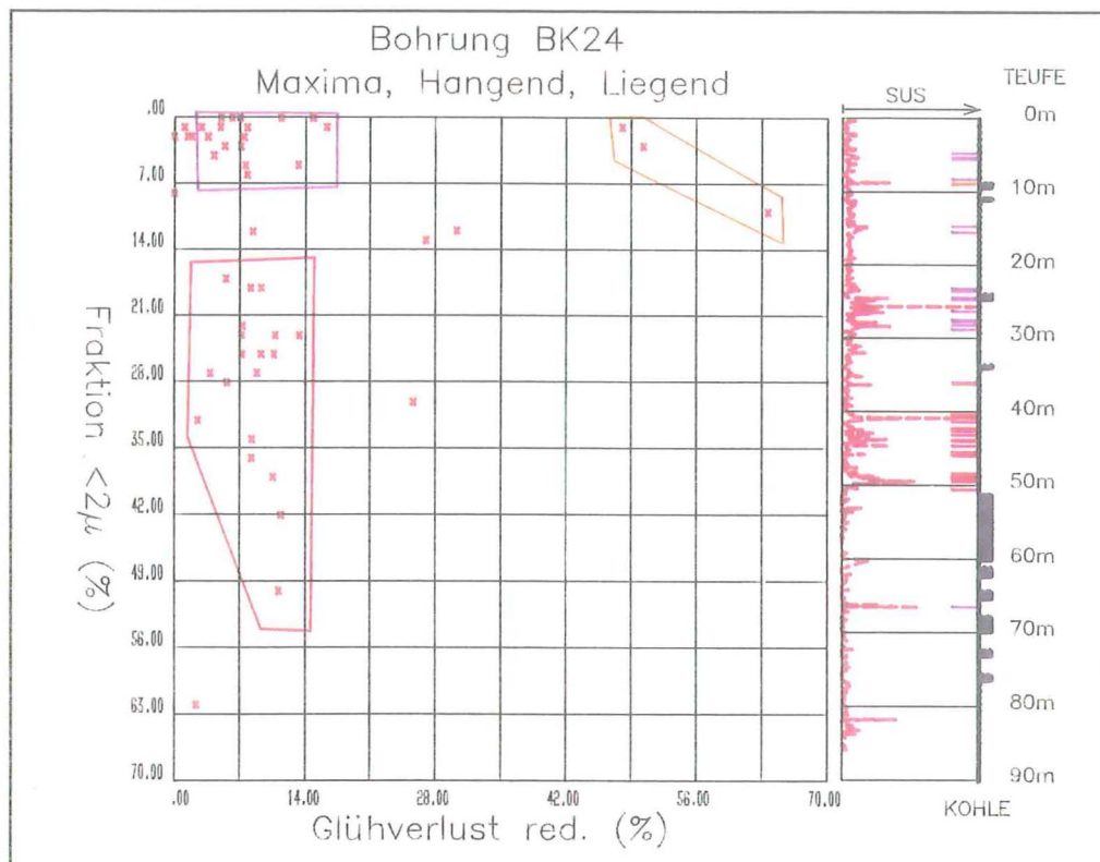
Abb.4b) Crossplot Glühverlust reduziert gegen Fraktion < 2µ erweitert durch Logdarstellung der Suszeptibilität
