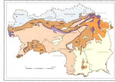
Tektonische Übersicht 1:2.000.000
