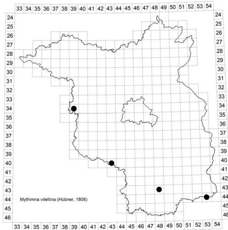
Abb. 2: Lage der bisher bekannt gewordenen Beobachtungen von Mythimna vitellina in Brandenburg.
