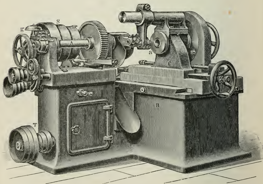
3. Rundfräsmaschine.
