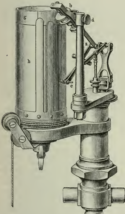
Fig. 3. Indikator von Dreper, Rosenkranz u. Droop mit Hamann's Planimeter-Vorrichtung.
