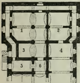
Fig. 1. Tresor. 1 Hauptkassette, 2 Urkundenraum, 3 Bankkassette, 4 Buchhalterei, 5 Packkammer und 6 Wächterzimmer.
