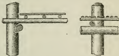
Fig. 1. Konstruktion der Plattform eines Hauses in Sarawak.
