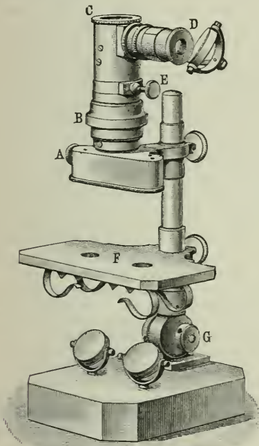
Fig. 1. Spektroskop von Zeiß.
