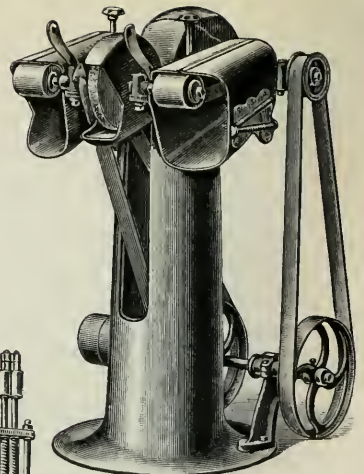
9. Sohlenabglasmachine.
