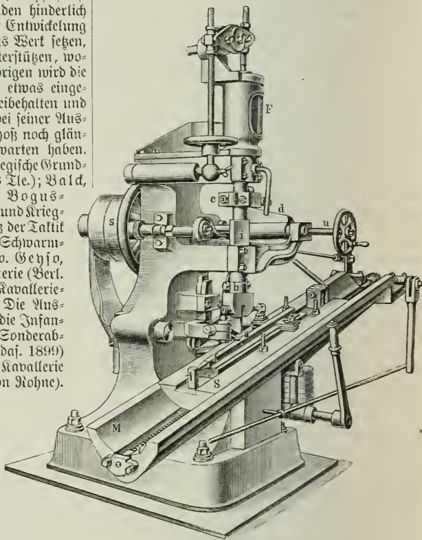
Fig. 1. Feilenhaumaschine.
