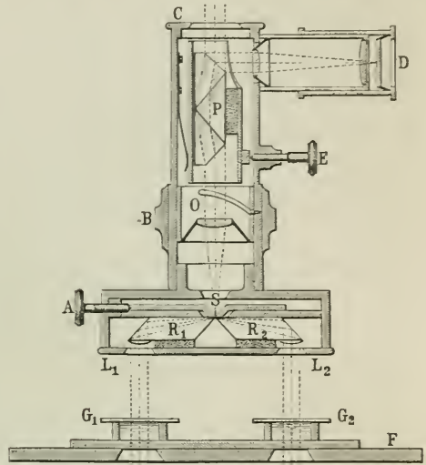
Fig. 2. Gang der Lichtstrahlen im Spektroskop.
