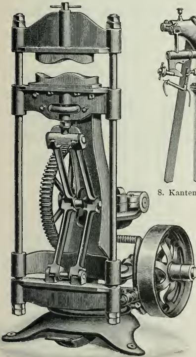
2. Sohlenformpresse.
