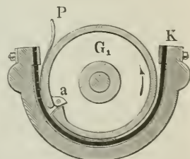
Fig. 2. Durchschnitt des Knitterapparats.
