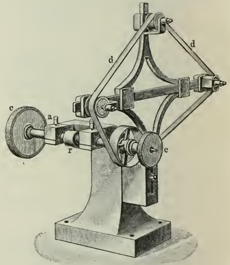
Schleifmaschine.
