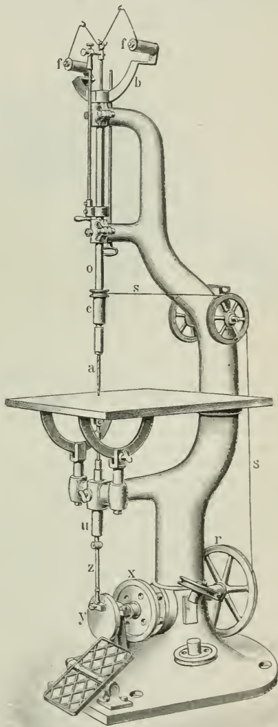
Fig. 1. Rotativsäge.
