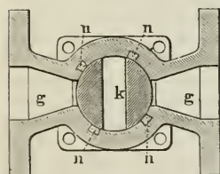
Fig. 2. Horizontalschnitt.
