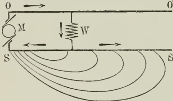
Fig. 2. Vagabundierende Ströme.
