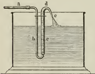
Fig. 4. Nitschescher Durchlüftungsapparat.
