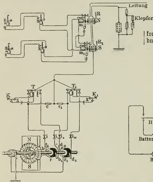
Fig. 1. Roberfons Vierfachsystem.
