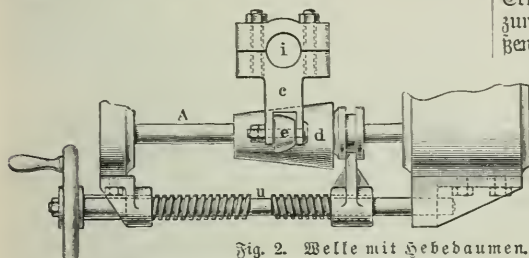
Fig. 2. Welle mit Hebebaumen.
