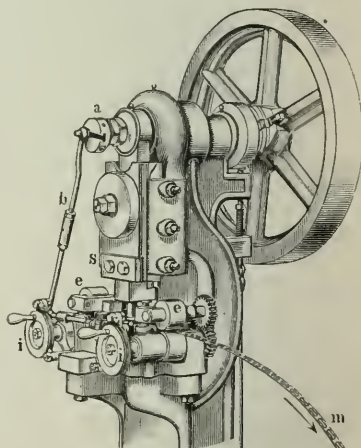
Fig. 3. Exzenterpresse zum Ausstangen.
