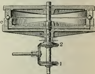
Fig. 3. Kugelschleifmaschine.
