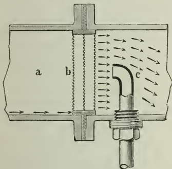
Fig. 2. Vorrichtung zur Entnahme von Dampfproben.
