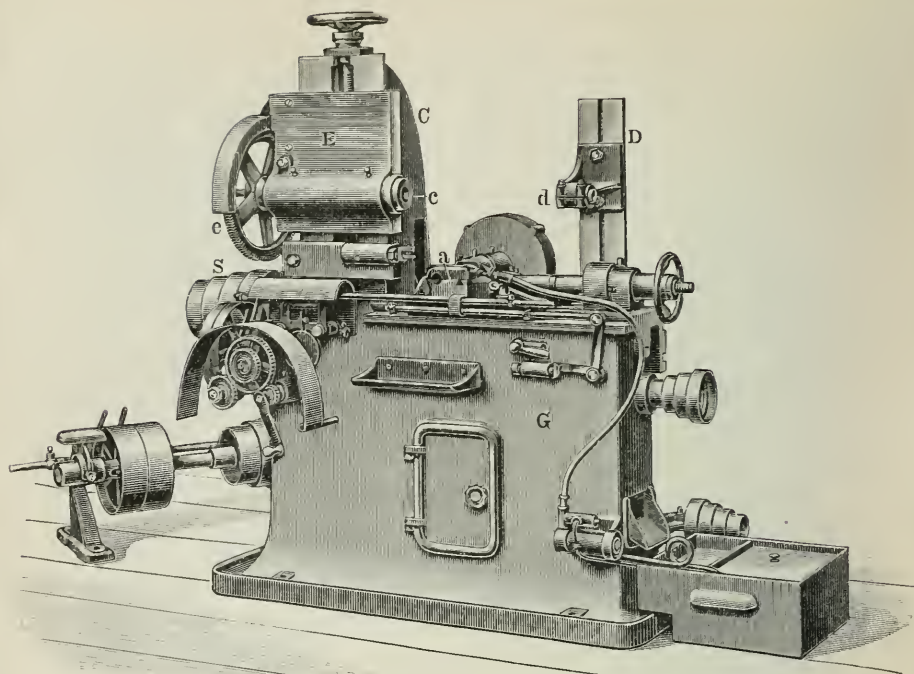
4. Selbstthätige Räderfräsmaschine.
