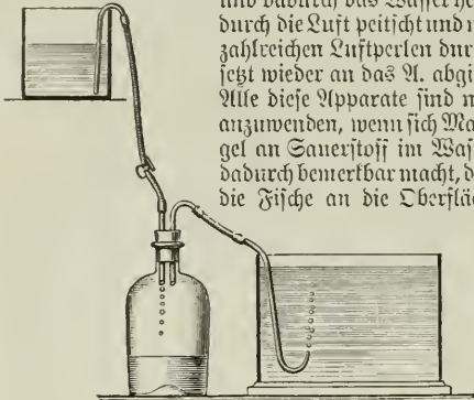
Fig. 3. Einfacher Durchlüftungsapparat.
