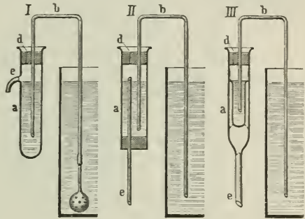
Fig. 2. Ablaufheber.
