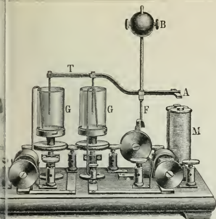
5. Foucaultscher Quecksilberunterbrecher.
