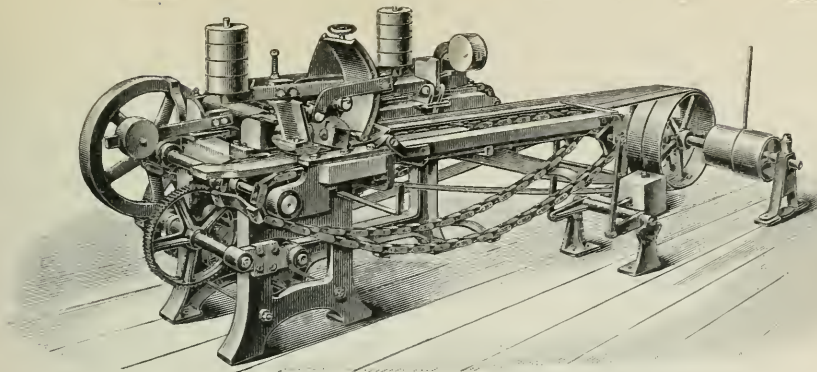
2. Daubenhobelmachine.
