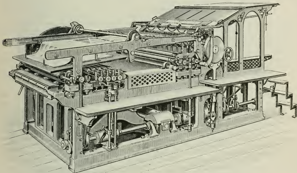
Fig. 1. Schnellpresse von König u. Bauer für Chromotypographie mit Frontbogenaustrag.
