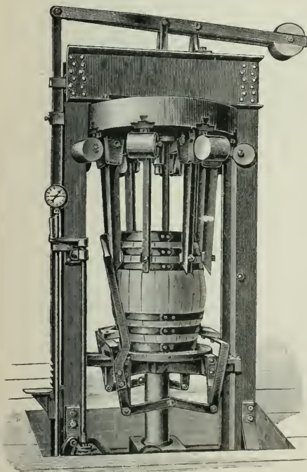
5. Reifenauftreibmaschine.
