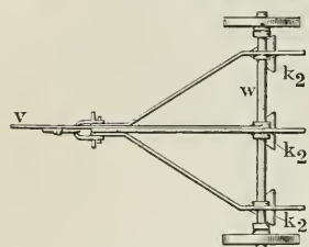
Fig. 3. Anker zum Befestigen der Kette.
