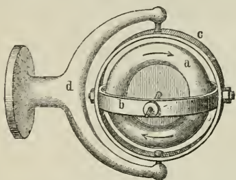
Fig. 1. Obrysches Gyroskop zur selbstthätigen Torpedosteuerung.
