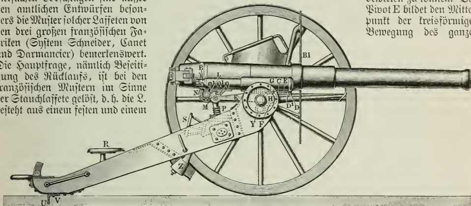
Laffete für Schnellfeuerfeldgeschütze von Maxim-Nordenfjelt.
