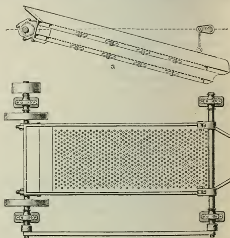
Fig. 2. Laues Tafelschwinggieb. a Seitenansicht.
