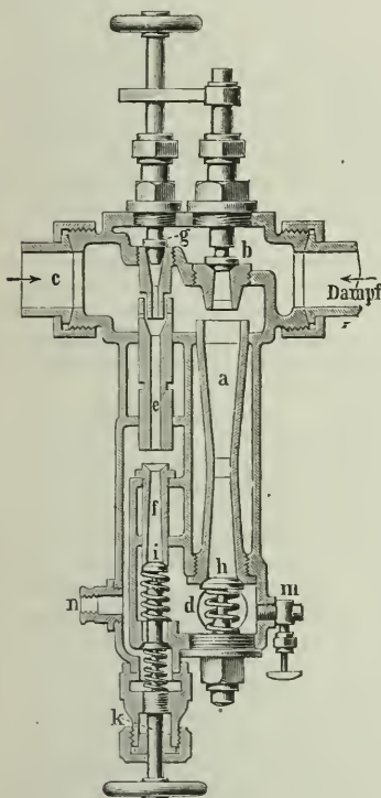
Nathans Dampfstrahlvorrichtung.
