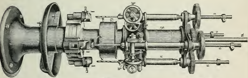
2. Vierspindelige Bohrmaschine.
