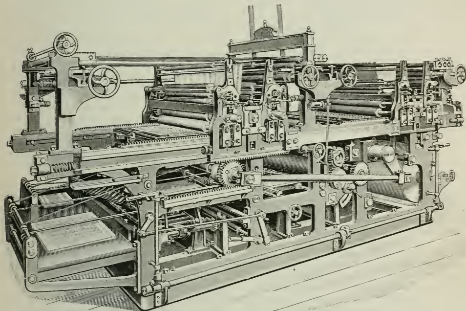
Fig. 2. Flachdruckrotationsmaschine von H. Hamm in Heidelberg und Frankfurt a. M.
