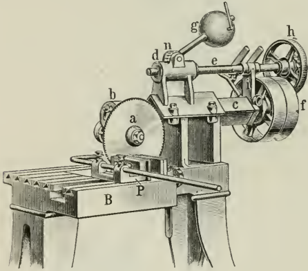
Fig. 2. Kältsäge.
