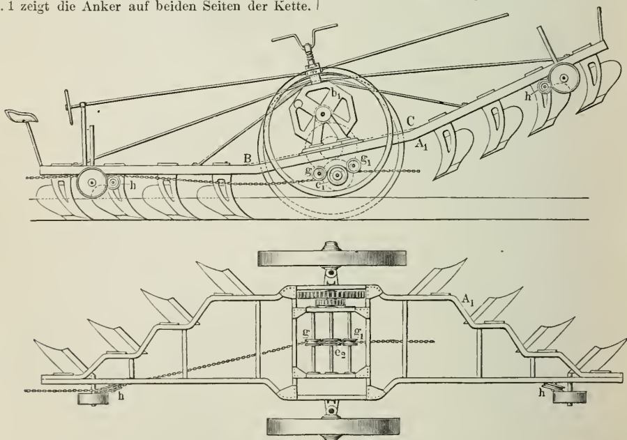
Fig. 4. Ansicht und Grundriß des Motorpfluges.
