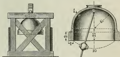
Appunns Viktoriaglocke. Ansicht und Durchschnitt.
