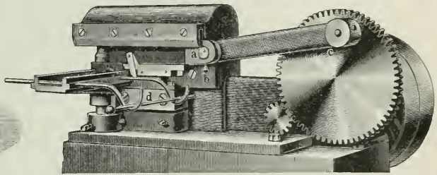
11. Speichengewinderollmaschine.
