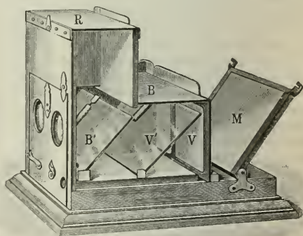
Fig. 5. Chromoskop, geöffnet.
