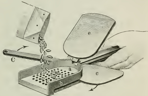
Pöhl's Kornprüfer bei der Füllung.
