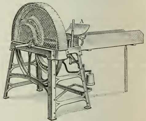
Häckselmaschine von Lanz.
