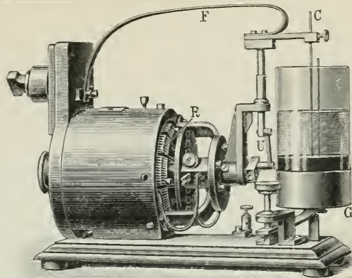
8. Motorquecksilberunterbrecher.
