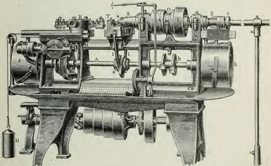
9. Selbstthätige Revolverdrehbank.
