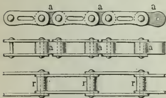
Fig. 16. Ketten.
