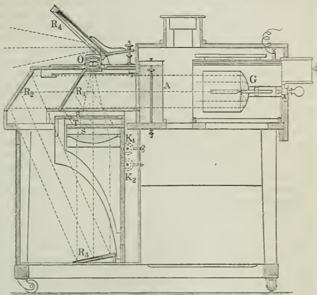
Epidiaskop von Zeiss.
