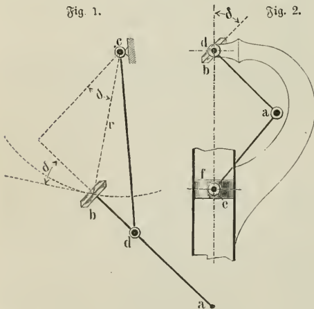
Fig. 1. Planimeter. Fig. 2. Hamanns Planimeters Vorrichtung für Indikatoren.
