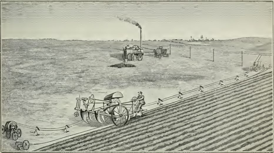
Fig. 1. Gesamtansicht des Motorpfluges von Fritsche und Pischon.
