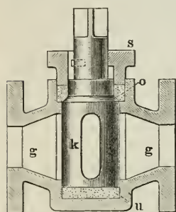
Fig. 1. Vertikalschnitt.
