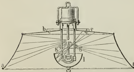
Fig. 2. Durchschnitt.
