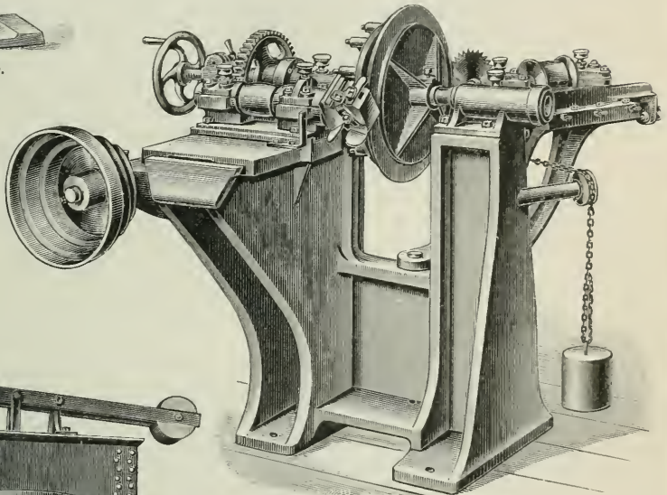
3. Bodenrundscheidmaschine.
