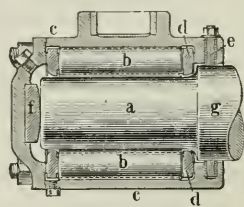
Fig. 2. Längsschnitt.
