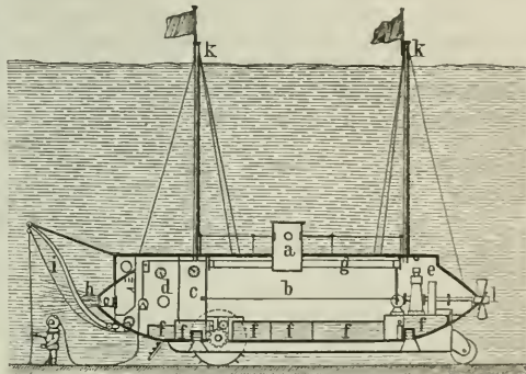
Unterwasserboot Argonaut.
