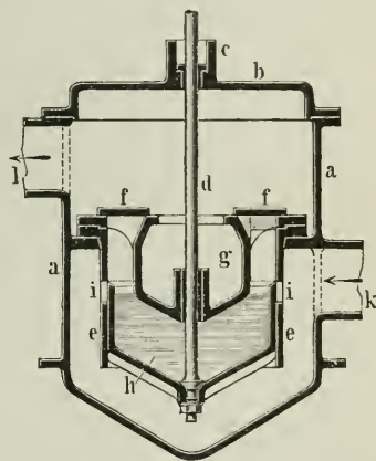
Stehende Luftpumpe ohne Saugventile.
