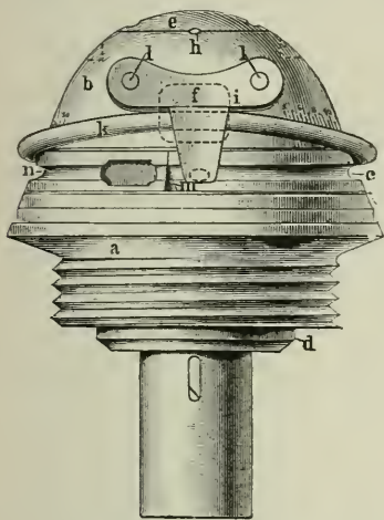
Doppelzünder für die Schnellfeuerkanonen der deutschen Feldartillerie.
