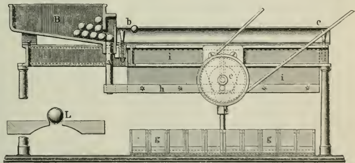
Fig. 6. Kugelfortiermaschine.
