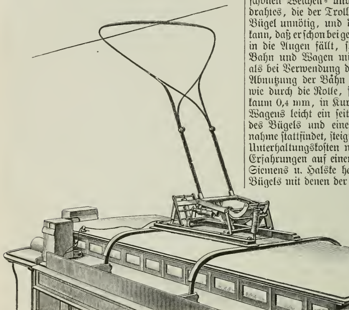
Fig. 1. Bügelschleifkontakt von Siemens u. Halske.
