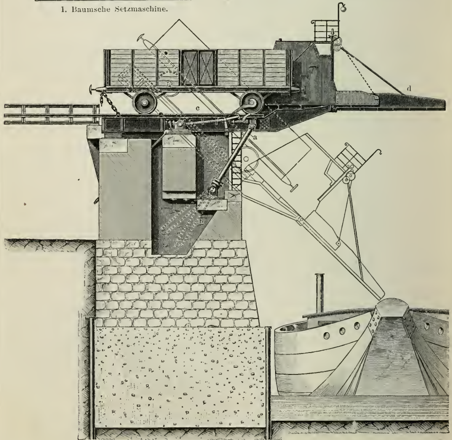
3. Kohlenkipper, System Schmitz-Rohde.
