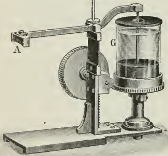
6. Quecksilberwippe.
