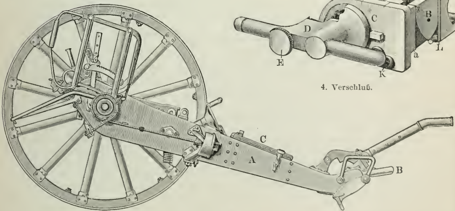
6. Die Feldlafete C/96.
