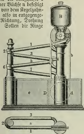
Fig. 4. Maschine zur Prüfung der Kugelform. a Obere Ansicht der ersten Schienen und Bogenstücke.
