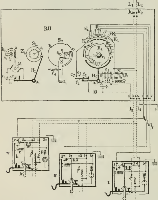
Fig. 11. Gemeinsame Fernsprechleitung für mehrere Teilnehmer, nach West.
