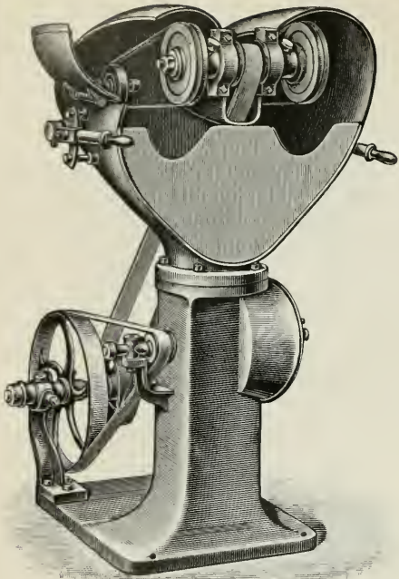
7. Absatzausglasmachine.
