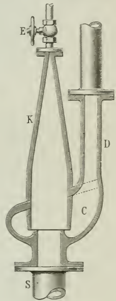
Fig. 2. Vertikalschnitt.
