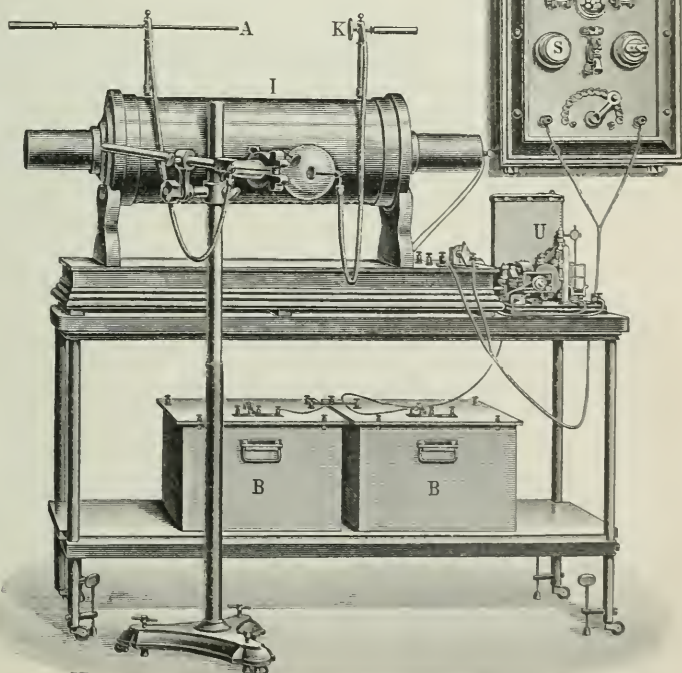
9. Röntgeneinrichtung mit Akkumulatorenbetrieb.
