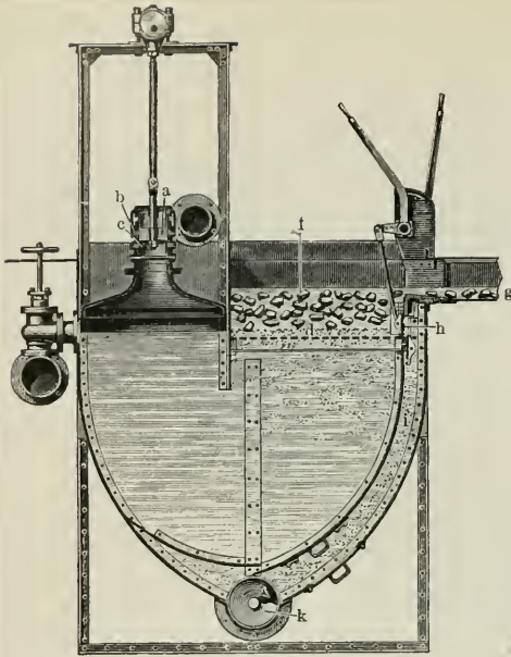
1. Baumsche Setzmaschine.
