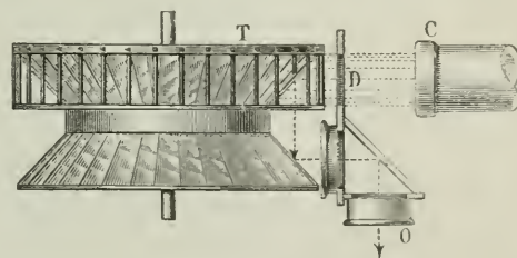
Fig. 4. Methorama. Grundriß.
