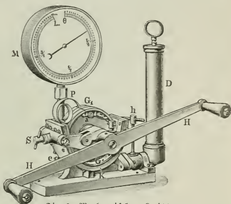
Fig. 1. Mechanischer Knitterer.
