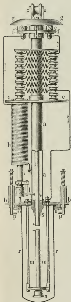
Conja=Dauerbrandlampe.
