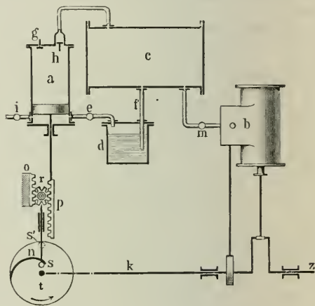
Benzinflufmotor von Durand=Noury.
