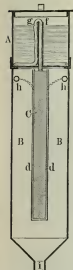
Fig. 1. Längsschnitt.
