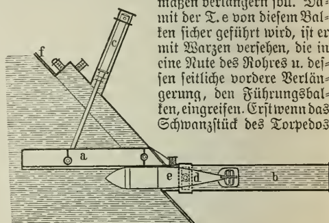
Fig. 2. Raselowitsky'sches Unterwasser-Breitseitrohr.
