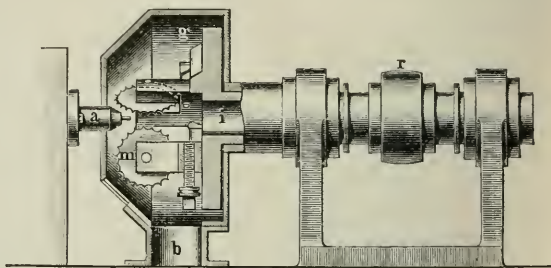
Fig. 1. Kugeldrehbank.
