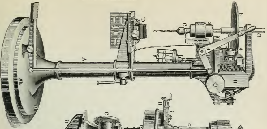
1. Schnellbohrmaschine mit elektrischem Antrieb.
