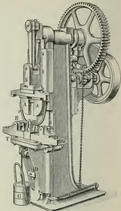
Fig. 2. Lentarmenpresse.
