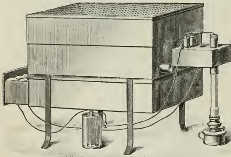
Fig. 2. Brütapparat von Schwarzlose.
