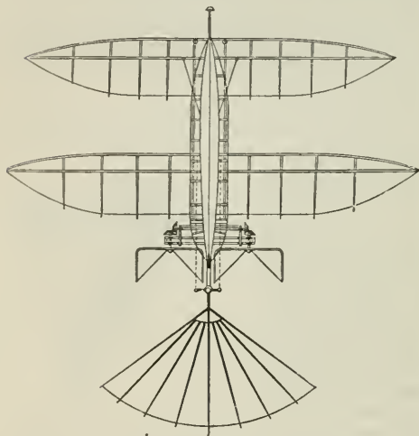
Fig. 2. Flugmaschine von Kress.
