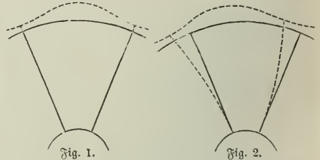
Fig. 1. Schwungrad unter dem Einfluß der Zentrifugalkraft ohne und mit gleichzeitiger Stoßwirkung.
