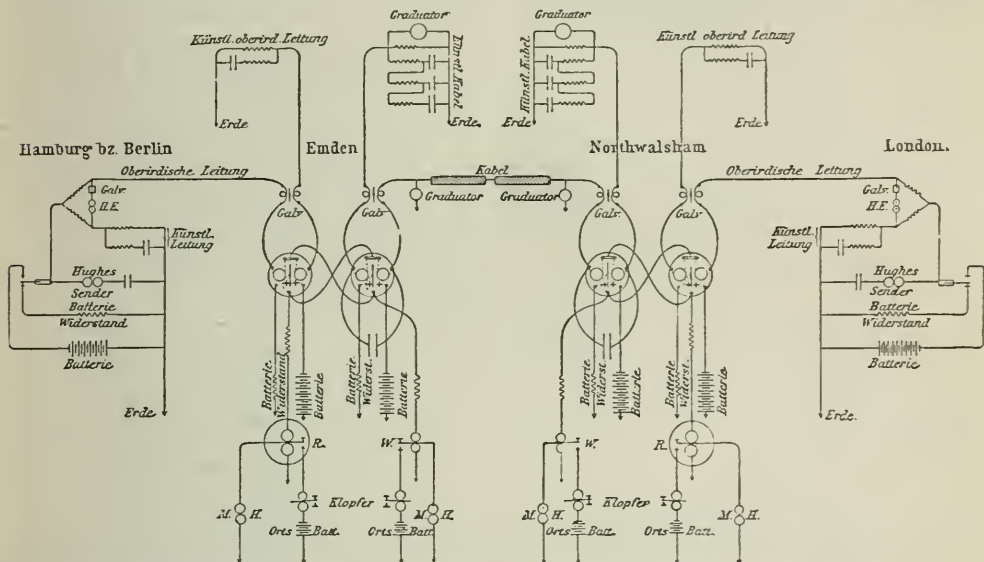
Fig. 3. Schaltung und Wirkungsweise der Übertragungsstationen des Hughes'schen Gegensprechers auf der Leitung Berlin-London. H. E. Hughes = Empfänger, M. H. Willeke = Hughes, R. Relais, W. Wheatstone.
