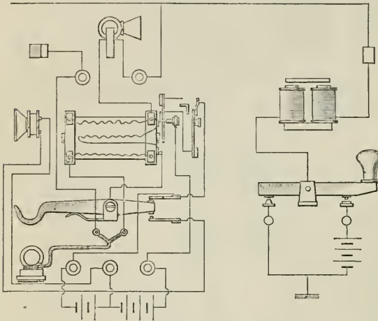
Fig. 4. Stromlauf beim Telegraphieren und Fernsprechen auf derselben Leitung.
