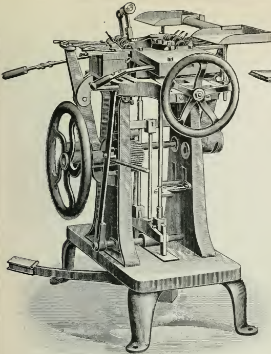
3. Chase, Aufzwickmaschine.
