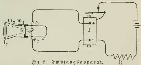
Fig. 2. Empfangsapparat.
