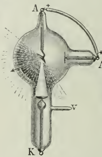
17. Röntgenröhre mit zwei Anoden.
