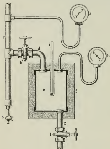
Fig. 1. Drosselkalorimeter von Peabody.
