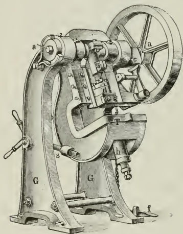
Fig. 1. Exzenterpresse.
