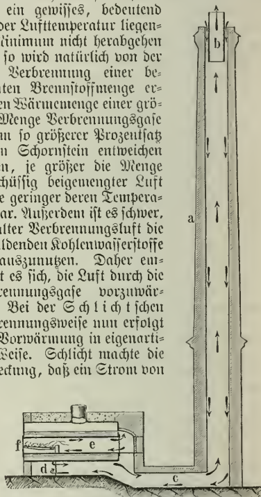
Feuerungsanlage nach Schlicht.
