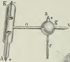
18. Regulierbare Röntgenröhre.
