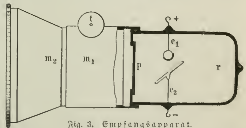
Fig. 3. Empfangsapparat.
