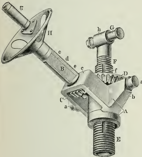
7. Richtmaschine.
