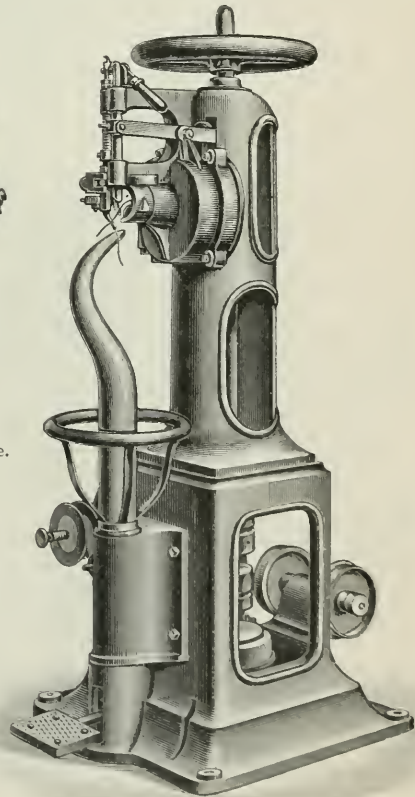
4. Allianz, Doppelsteppstich-Sohlennähmaschine.
