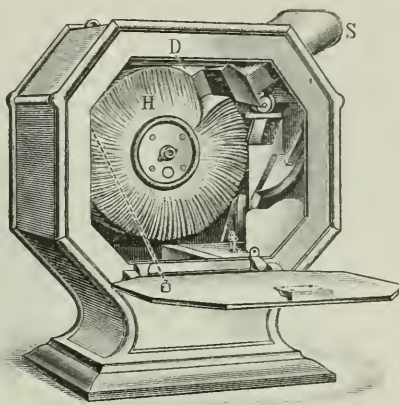
Fig. 1 u. 2. Mutoskop.
