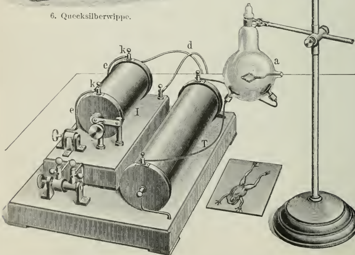
11. Röntgeneinrichtung mit Teslatransformator.
