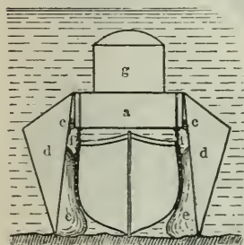
Fig. 4. Hebekörper von Clarf u. Stanjfeld.
