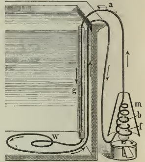
Fig. 5. Heizapparat.
