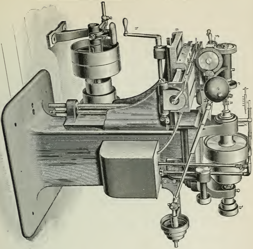
5. Tabellkreuzfräsmaschine.
