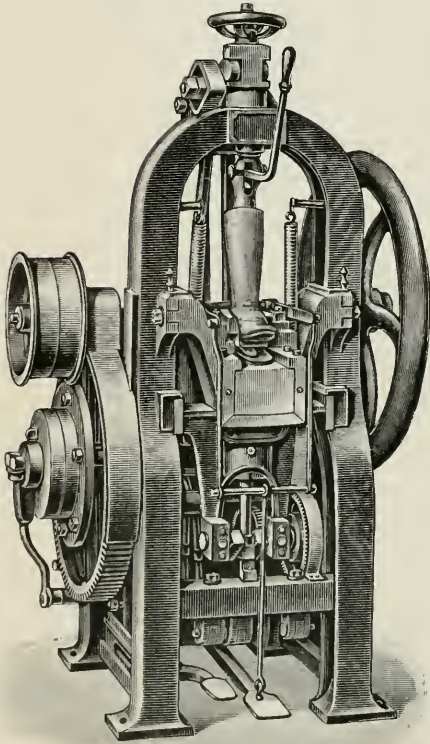
6. Perfecta, Absatzpreß- und -Aufnagelmaschine.
