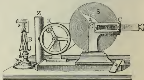
Fig. 1. Scheiners Sensitometer.
