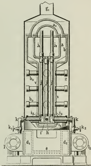
Fig. 2. Ätherdampfmaschine von Rhodes.
