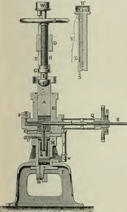
Zementprüfungsmaschine von Amster-Laffon.
