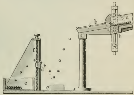
Fig. 5. Härteprüfer.
