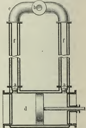
Fig. 3. Ammoniaksalzmotor von Pape (Längsschnitt).
