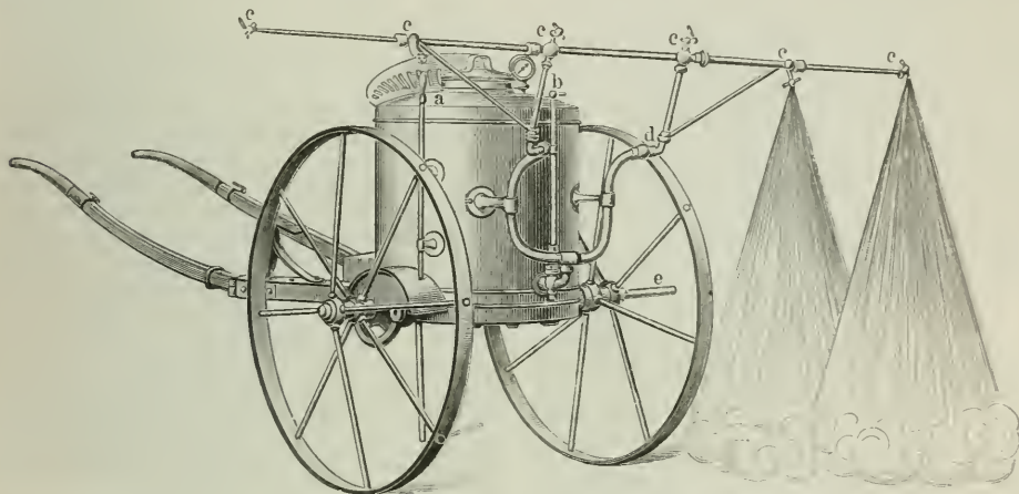
Fig. 2. Fahrbarer Peronospora-Apparat.
