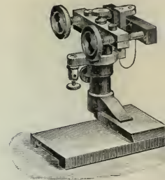
4. Platinunterbrecher nach Deprez.
