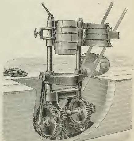
6. Reifenziehmaschine.
