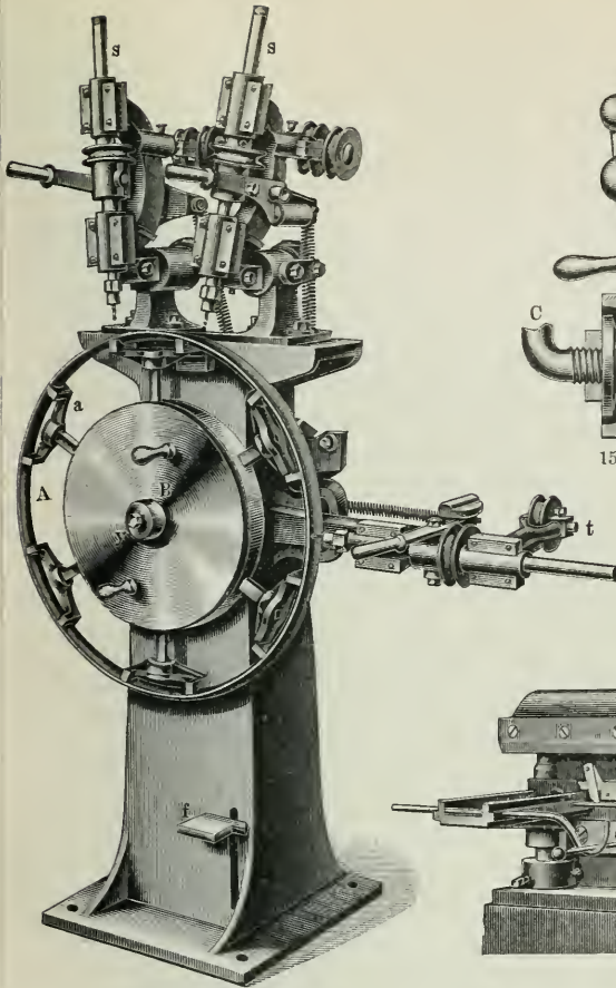
14. Felgenbohrmaschine.
