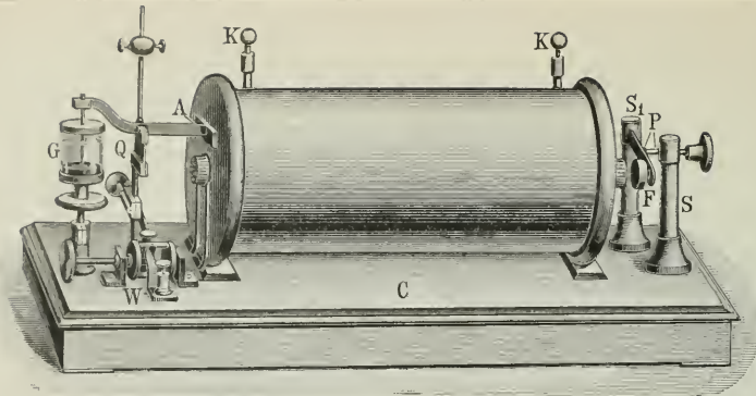
3. Kleines Funkeninduktorium mit Quecksilberwippe, Wagnerschem Hammer, Kondensator und Stromwender.
