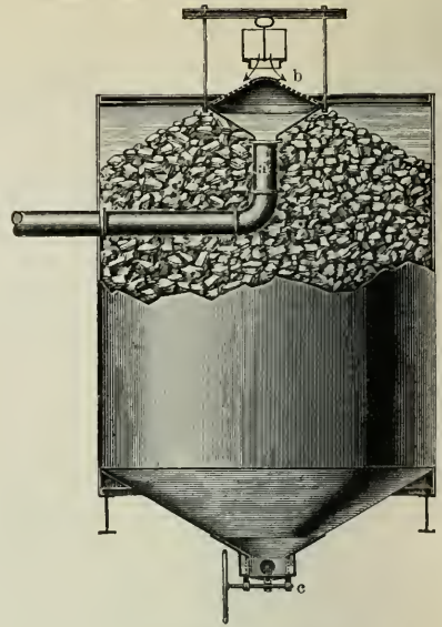
2. Verladetasche für Nußkohlen, System Baum.
