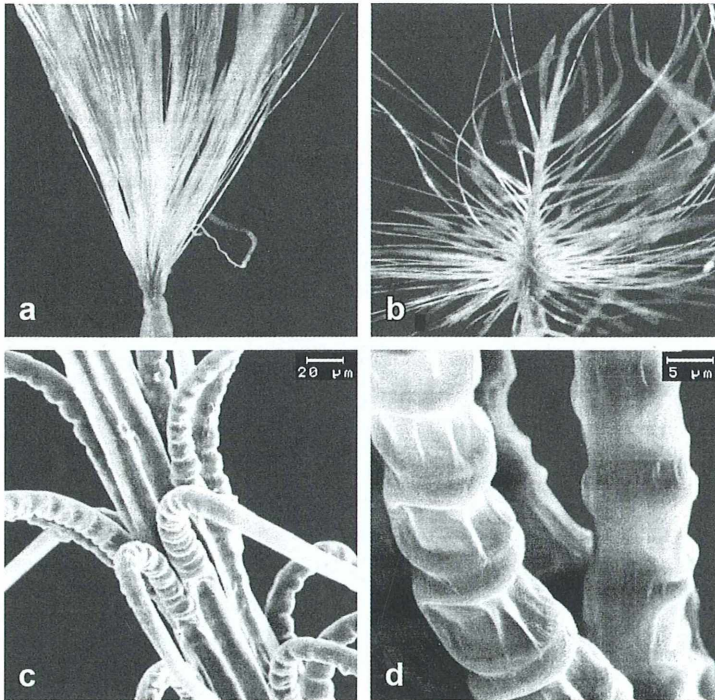
Abb. 2: Biologische Krümmungs-Verstelleinrichtung mit hygroskopischen, seriellen Elementen an der Basis der Pappus-Haare der Diaspore von Tamarix gallica . a, b Makro, kurz nach Entnahme aus der Feuchten Kammer (a) und 30 s danach (b) bei circa 60% relativer Luftfeuchte. c, d Rasterelektronenmikroskopie (REM) (vollständig getrocknet). c Biegeebenen an der Basis einiger Flughaare. d Einzelne Biegeebenen. REM-Aufnahmen A. Wissner, Saarbrücken.
