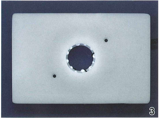
Abb. 2: Fertig montierter Grundkörper aus schwarzem POM (Polyoxymethylen) mit eingesetztem LED-Ring fertig verdrahtet. – Abb. 3: Ansicht mit aufgelegter Tischplatte.
