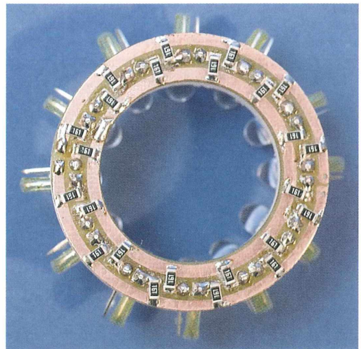
Abb. 4: Platinenseite des LED-Ringes mit SMD-Widerständen (SMD = surface mounted device).
