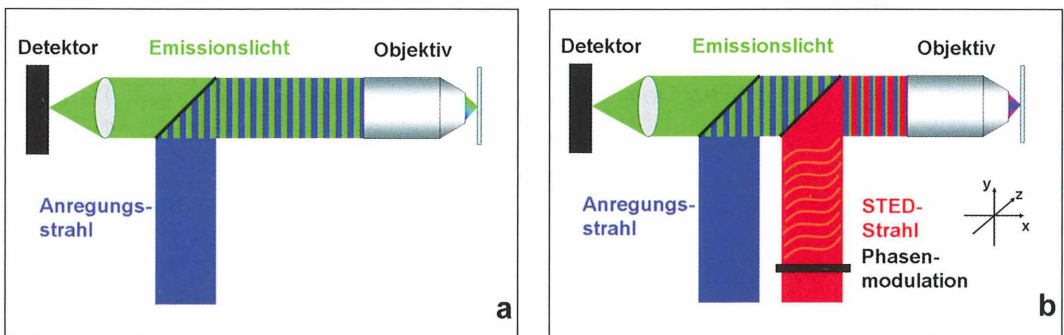
Abb. 2: Die linke Abbildung (a) zeigt schematisch den Aufbau eines Laserscanningmikroskops. Der Anregungsstrahl (blau dargestellt) wird über einen teildurchlässigen Spiegel in den Strahlengang des Mikroskops eingekoppelt und erreicht durch das Objektiv das Objekt. Der Brennfleck des Anregungslichtes hat beugungsbedingt einen Durchmesser von etwa gut 200 nm. Das blaue Licht regt Fluoreszenzmarker, die an Organellen oder Molekülen in der Zelle gekoppelt sind, zu grüner Fluoreszenz (Emission) an. Nachteil: Objekte, die näher als 200 nm beieinander liegen werden nicht getrennt dargestellt, sondern verschmelzen in der Abbildung zu einer unscharfen Masse. In der STED-Mikroskopie (b) wird ein zweiter Laserstrahl, der Abregungsstrahl (rot), zeitlich synchronisiert ebenfalls über einen speziellen Spiegel in den Strahlengang eingekoppelt. Der rote Abregungsstrahl ist ringförmig und überlagert den Brennfleck des grünen Anregungsstrahls. Dadurch wird die Fluoreszenz in der Peripherie des Brennflecks ausgeschaltet. Zur Fluoreszenz kommt es nur noch im „Loch des Doughnut“. Je höher die Intensität des roten Abregungsstrahls ist, desto kleiner wird der Brennfleck des Anregungslichts und die Auflösung steigt (Abbildungen: Max Planck Gesellschaft, Berlin).
