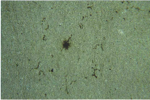
Abb. 3: Solnhofener Plattenkalk; feinkörniger Kalkstein.
