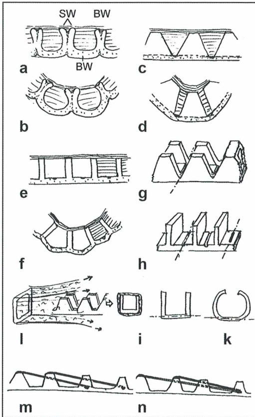
Abb. 4: Schemata der Wirkungsweise der hygroskopischen Krümmungs-Verstelleinrichtung an der Flügelhaarbasis von Tamarix gallica (a, b) und bionisch-technische Abstraktionen (c–n), bei feuchter Luft (a, c, e) und bei trockener Luft (b, d, f). Bei f links nur Decken-Zugband aus hygroskopischem Material, rechts zusätzlich auch Seitenbänder. Seitansichten. Elastische Basiswand BW punktiert, Seitwände SW hell, hygroskopische Membran liniert. g, h Blockdiagramme möglicher Trägereinrichtungen; Biegeachsen strichpunktiert, g, h links Kerbe, rechts Langloch; h entspricht e. i, k Querschnitte möglicher Trägereinrichtungen, Biegeachsen strichpunktiert. l Überziehen einer Trägereinrichtung mit einer aus einer Ringdüse austretenden, aufschumpfenden und/oder aufklebenden hygroskopischen Membran. m, n Hygroskopisch aktive Spannbänder, die über mehrere Elemente zu unterschiedlichen Punkten (m) oder zu einem Punkt (n) führen.
