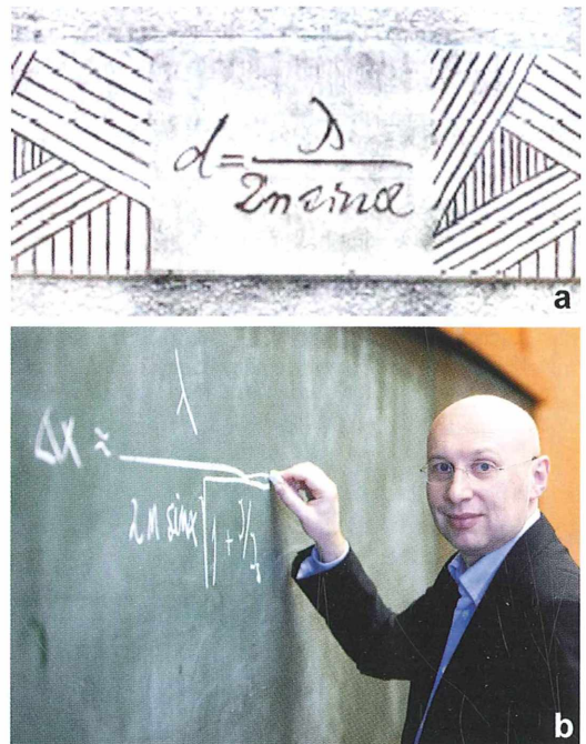
Abb. 1: a In Jena in Stein gemeißelt: Die Abbe'sche Auflösungsformel: d = \lambda / 2n \sin \alpha . Sie war 130 Jahre lang ein unumstößliches Gesetz. Doch Stefan Hell brach das Gesetz und schrieb diese Formel neu (b): von der Abbe'schen Formel zur Hell'schen Formel (Fotos: a Deutscher Zukunftspreis, 2006, Pressemitteilung; b Ansgar Pudenz, Deutscher Zukunftspreis).
