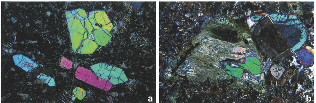
Abb. 5: Alteration von Olivin in vulkanischem Gestein (XPL-Beleuchtung). a Frische Olivinkristalle. b Umwandlung von Olivin in Serpentin; nur ein kleiner Kern (grün) ist unverändert geblieben. Die Umwandlung betrifft lediglich die Olivine; der Augitkristall (blau) rechts erscheint völlig unangegriffen.
