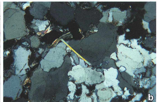
Abb. 4: Buntsandstein. a LPL-, b XPL-Beleuchtung. Das Gestein enthält neben Quarzkörnern wenige Glimmerplättchen (in der Bildmitte ein Muskovit), ansonsten noch etwas feinkörnige Matrix. Bei der Gesteinsdiagenese ist Quarzzement an den Sandkörnern angewachsen. Die ursprünglichen Korngrenzen sind als feine Bänder von an der ehemaligen Oberfläche abgelagerter Matrix erkennbar.
