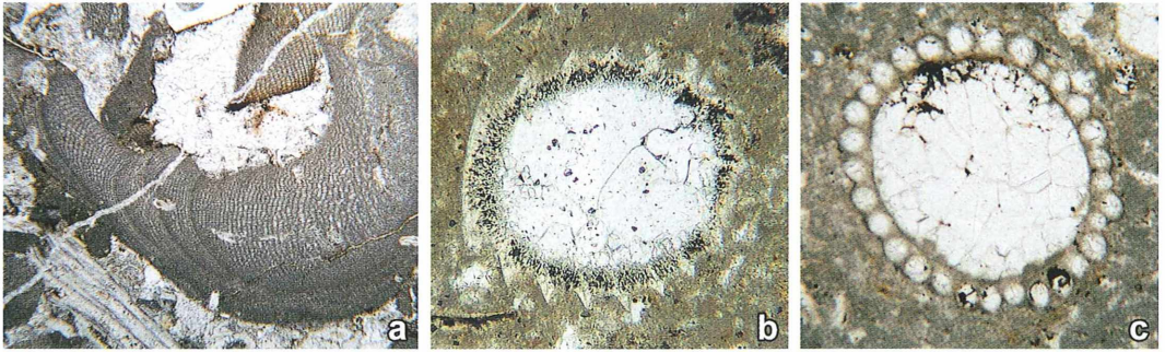
Abb. 2: Algenfossilien. a Lithothamnium sp., Längsschnitt durch Algenstock. b Chara sp., Längsschnitt durch Oogonium. c Chara sp., Querschnitt durch Trieb, die Rindenzellen sind deutlich erkennbar.
