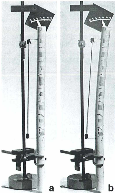
Abb. 5: Demonstrationsmodell. Bestehend aus einem PVC-Rundrohr (Durchmesser 2,5 cm, Höhe 50 cm), eingeschnitten nach Abbildung 4g, k (wegen der ungenügenden Eigenelastizität des Materials mit Rückhol-Spanngummi) und überklebt mit einer Zellophan-Folie (wegen der mäßigen Hygroscopie des Materials nur geringe Abbiegungen). a Bei 75% relativer Feuchte. b Bei 50% relativer Feuchte.
