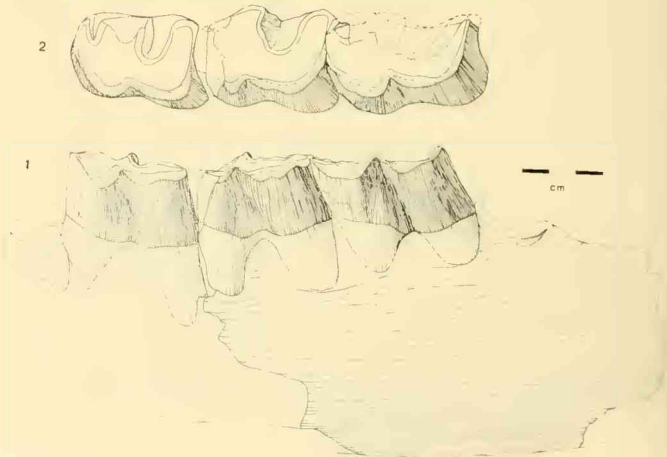
Abb. 1: Unterkieferbruchstück mit P_4 — M_2 li. Bayer. Staatsslg. Paläont. hist. Geol. Nr. 1926 X 2. Miozän, Langental, Südwestafrika. Ansicht von der Labialseite.
