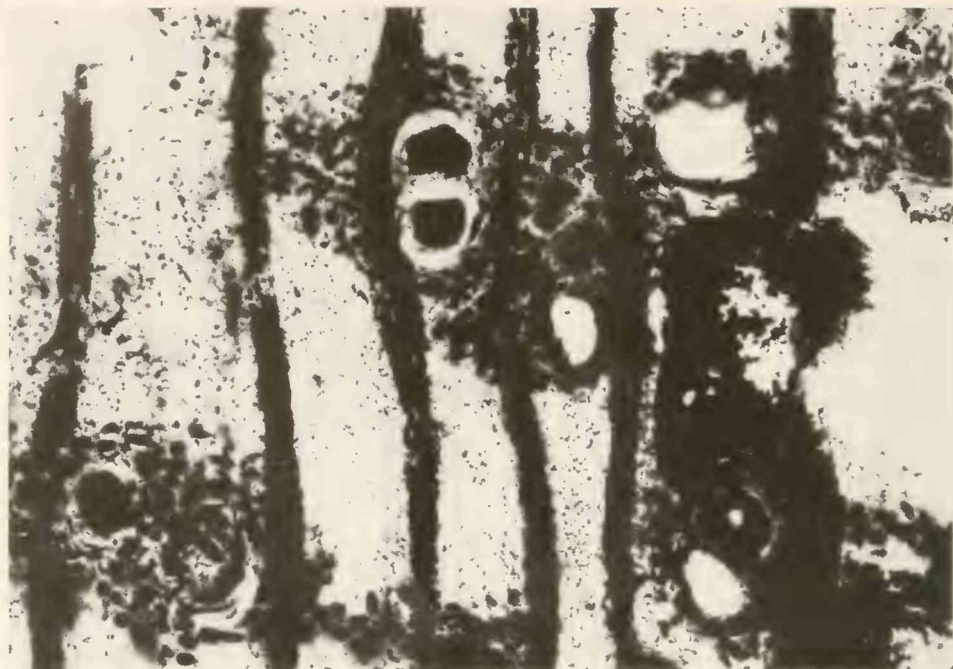
Abb. 5: Querschnitt. Dickwandige Gefäße, Parenchym vasizentrisch, schwach aliform, teils confluent. Inventar-Nr. BSP 1971 I 57. \times 150 .
