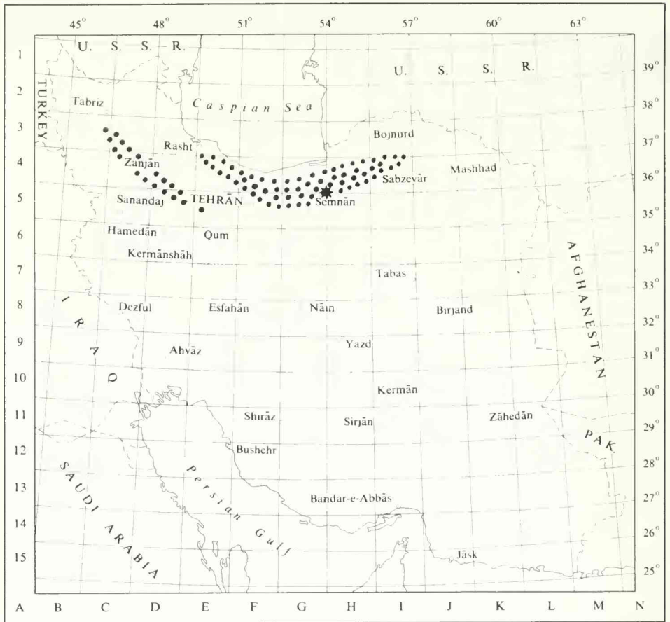
Abb. 1: Die Verbreitung der Dalichai-Formation (punktiert) und die Lage von Gardaneh-Ahovan (Sternchen), ca. 60 km E Semnan.
