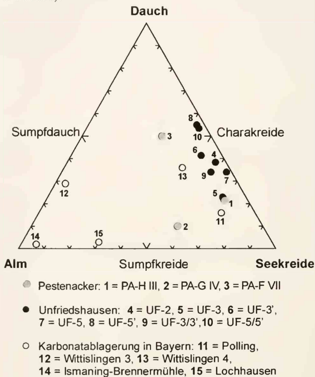
Abb. 6. Haupt- und Übergangstypen der quartären Binnenwasserkalke und ihre Ostrakodenfauna (nach ABSOLON 1974: Abb. 8).
