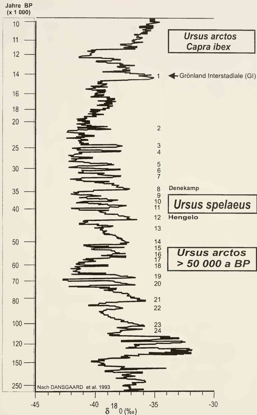
Abb. 2: Sauerstoffisotopenkurve ( ^{18}\text{O}/^{16}\text{O} ) des GRIP Eisbohrkernes (nach DANSGAARD et al. 1993). Darin dargestellt die zeitlichen Positionen der Fauna aus der Neuen-Laubenstein-Bärenhöhle. Graphik Rosendahl
