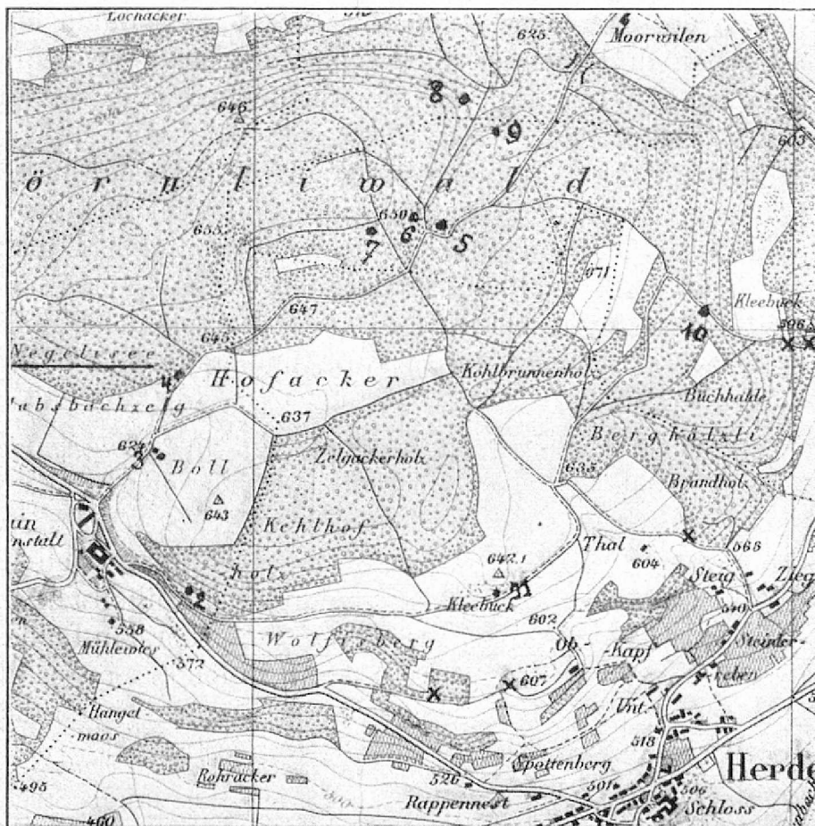
Fig. 2. Entblößungen des jüngeren Deckenschotter im Hörnliwald (Kalchrain-Herdern). Ziffern entsprechen dem Text. \times = miocäne Nagelfluh. (Top. Atlas 1 : 25 000, Bl. 56.)
