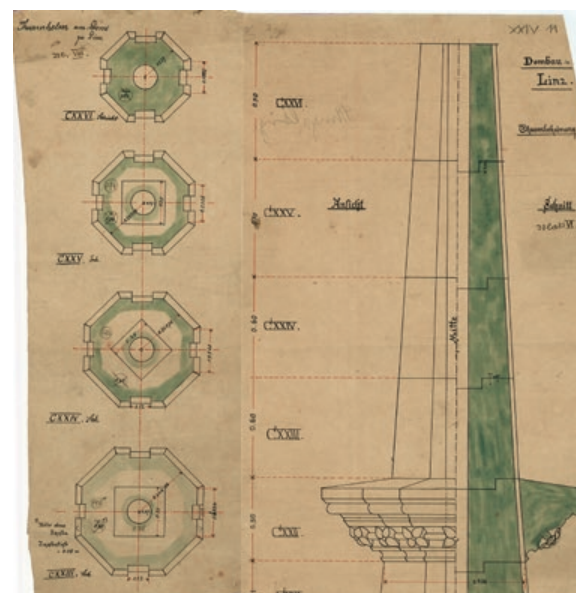
PLAN DES TURMHELMS UND DER TURMBEKRÖNUNG MIT EINGEZEICHNETEN STEINNUTEN UND -FUGEN.
