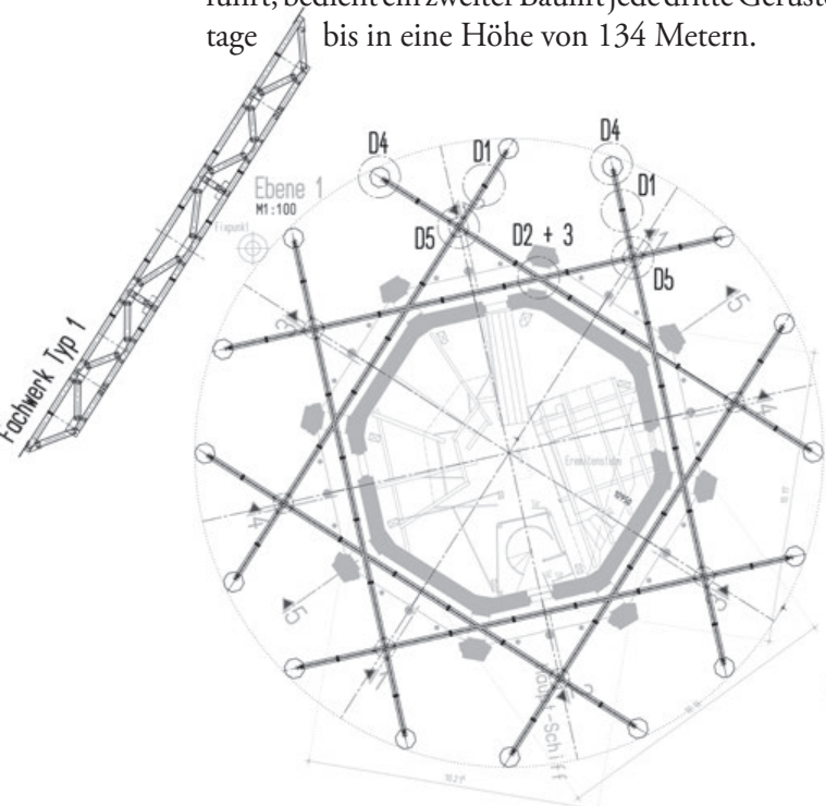
PLAN DER ZU ERRICHTENDEN STAHLFACHWERKKONSTRUKTION ZUR DURCHFÜHRUNG DER SANIERUNGSARBEITEN IN 65 METERN HÖHE.
