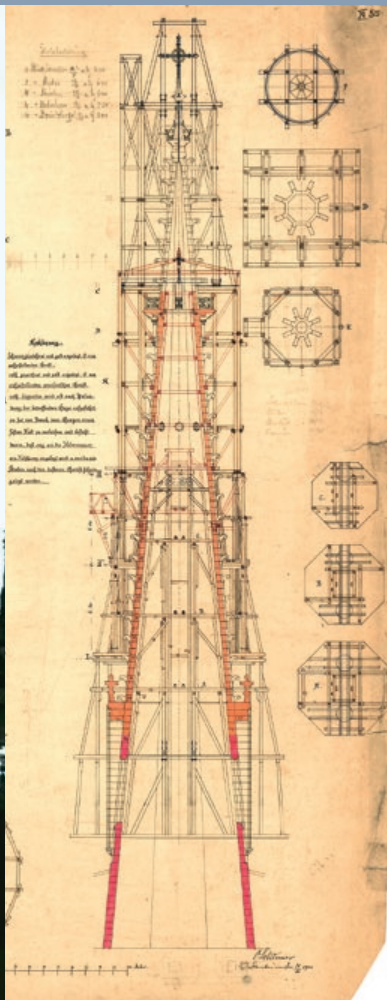
PLAN DES GERÜSTS ZUR ERRICHTUNG DES TURMHELMS.
