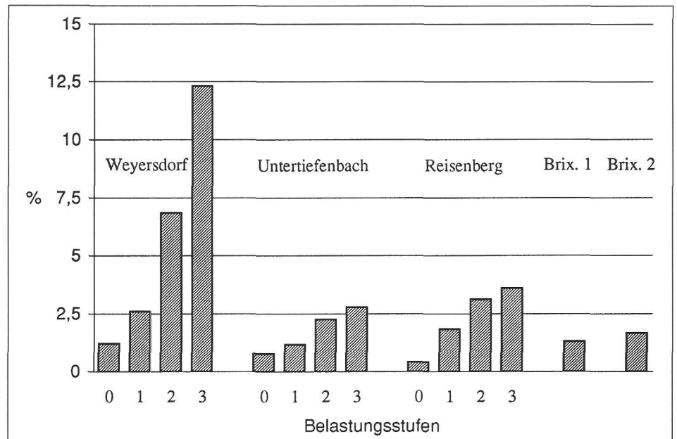
Abb. 5 Ammoniumacetat-lösliches Zink in % der gesamtsäurelöslichen Fraktion (Königswasser).
