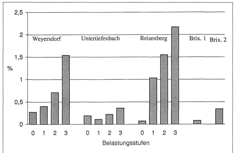
Abb. 4 Ammoniumacetat-lösliches Vanadium in % der gesamtsäurelöslichen Fraktion (Königswasser).
