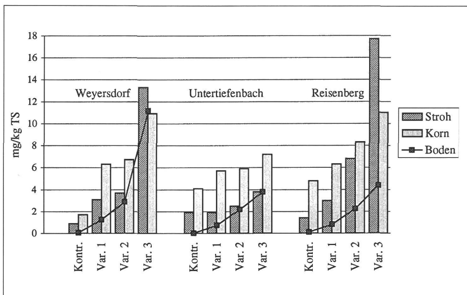
Abb. 7 Cu-Gehalte in Sommerweizen (Korn, Stroh) und in Ammonium-Acetat- Auszügen der Versuchsböden / Pro- ben 7/92.
