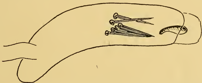
Abb. 1. — Aedoeagus von Peronea hastiana (L.) ab. combustana Hb. mit 6 Cornuti. — Präparat Nr. M. 225 (Lohr a. Main, coll. L. Osthelder).
