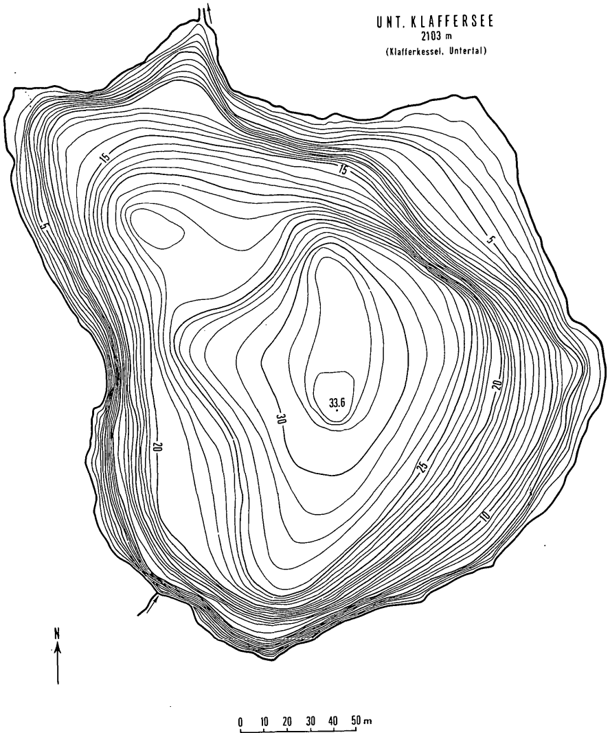
Abb. 9: Der Untere Klaffersee im Klafferkessel (2103 m).
