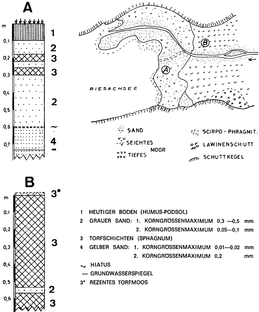
Abb. 23: Die beiden ergrabenen Profile im Verlandungsgebiet des Riesachsees, A 20 m und B 150 m vom See entfernt. A liegt im Raume der ehemaligen fluvialen Verschüttung. Horizont 4 erscheint durch eine ältere, vollkommen abgetragene Bodenbildung verändert worden zu sein; die Grenze zur oberen Schicht ist auch durch einen Wechsel in der Korngrößenhäufigkeit gekennzeichnet. Profil B liegt in einem Raum, der überwiegend biologisch verlandet ist, wobei man auf Grund der Lage annehmen kann, daß der Riesachbach durch einen ehemaligen Deltavorbau einen flachen Teil des Sees abschnürte (s. Lageskizze). Nur selten wurde das Torfwachstum ( Sphagnum sp.) durch Sandeinschüttungen unterbrochen.
