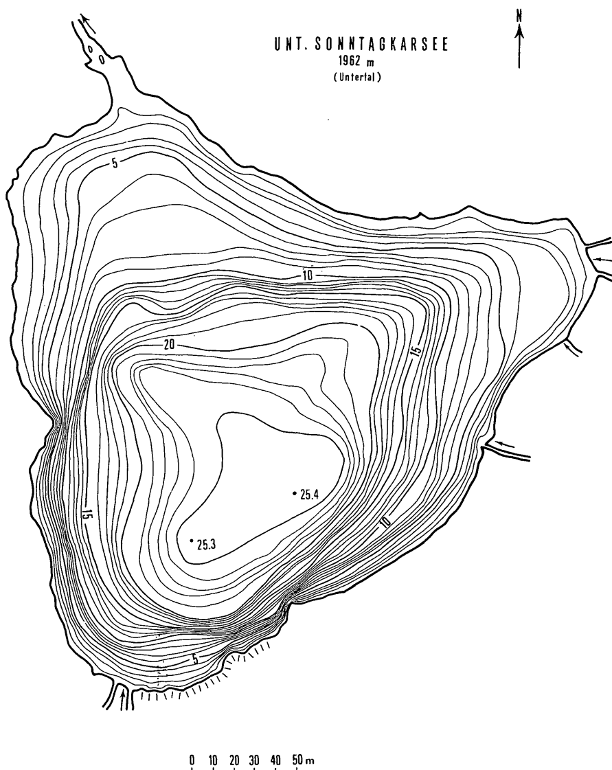
Abb. 5: Der Untere Sonntagkarsee im Riesachtal (1962 m).
