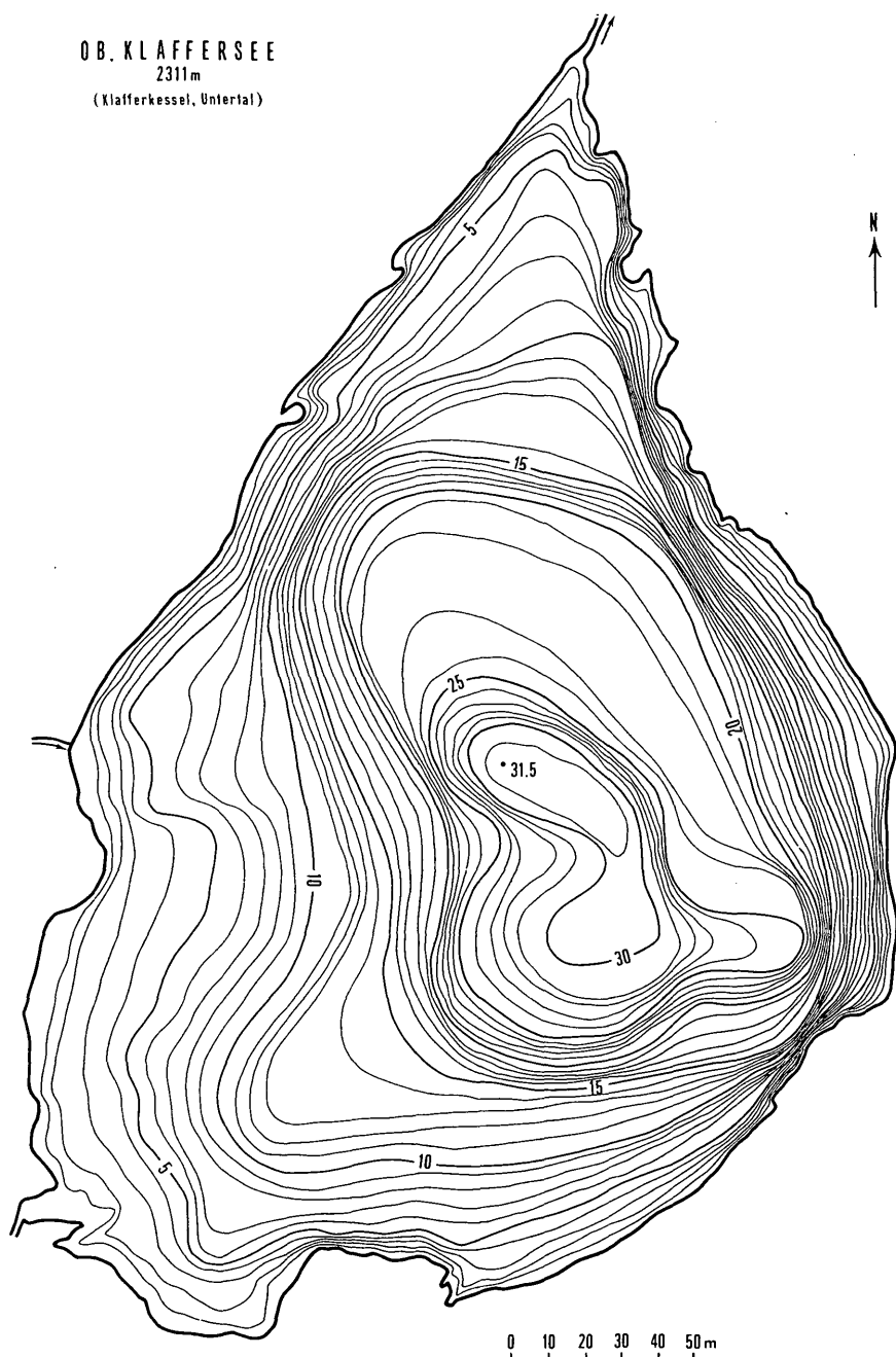
Abb. 13: Der Obere Klaffersee im Klafferessel (2311 m).
