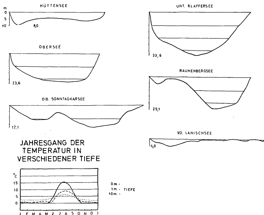
Abb. 20: Charakteristische Seepprofile, jeweils in W—E-Richtung durch die tiefste Stelle bei einer Überhöhung von ca. 1,5. Temperaturdiagramm verschiedener Wassertiefen am Riesachsee (Mittel 1969 und 1970). Die dick ausgezogene 0°m-Linie entspricht der Eisdeckenandauer.
