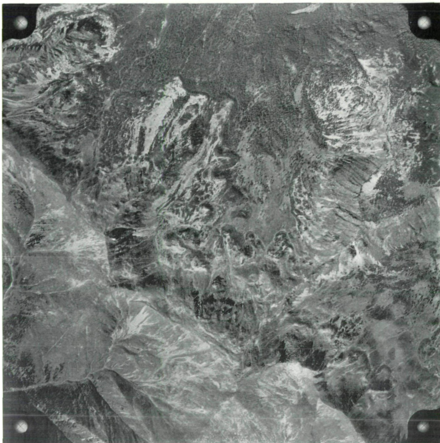
Abb. 9: Luftbild des Typs 1 „Brandstätter Kar“. Neben der starken Aufgliederung in einzelne Lappen ist deutlich der zentrale, ehemals gewölbte Stromstrich des Blockgletschers zu erkennen, der im Daunstadium eine neuerliche Aktivierung erfahren hat; am Rand gegen die Kämme sind postglaziale Schneeschuttwälle zu erkennen. Kammhöhe 2100—2200 m, Blockgletscherende ca. 1860 m. Verv. m. Gen. des Bundesamtes f. Eich- u. Vermessungswesen (Landaufnahme) Wien G. Z. L. 62.674/57.
