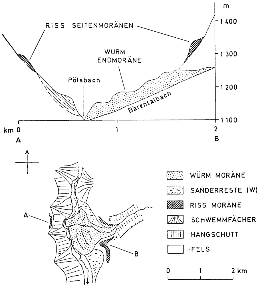
Abb. 5: Die Moränenlandschaft „Leitschacher“ am Ausgang des Bärentals ins Pölstal. Gut erhaltene Riß- und Würmmoränen.
