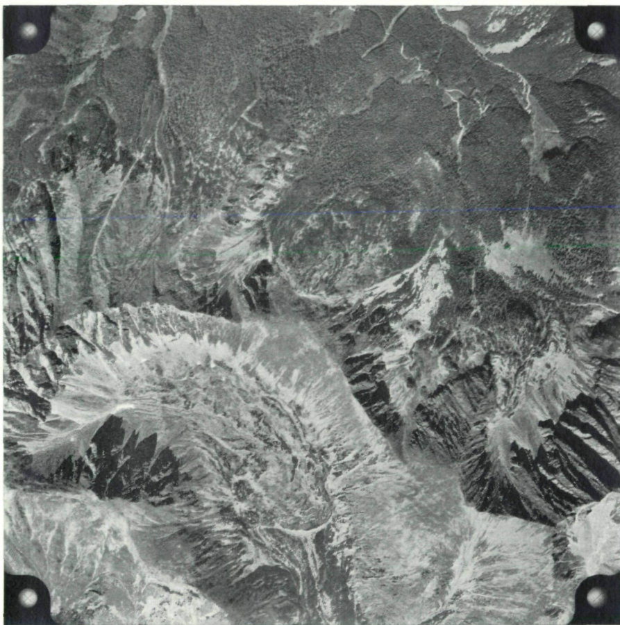
Abb. 10: Luftbild des Typs 3 „Hölltag“. An. linken Bildrand das Geierhaupt (2417 m). Neben dem gewaltigen Blockgletscher sind kleinere Formen nördlich des Kammes und die Asymmetrie der Bergrücken durch die Glatthangbildung und Karwandunterschneidung zu ersehen, Verv. m. Gen. d. Bundesamtes f. Eich- u. Vermessungswesen (Landesaufnahme Wien G. Z. L. 62.674/57.
