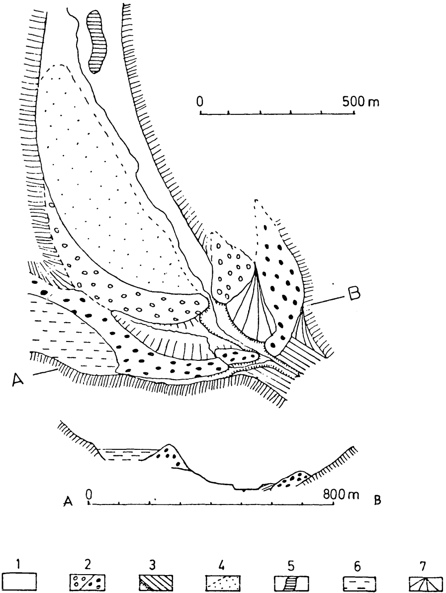
Abb. 6: Das Zungenbecken des würmzeitlichen Gaalgletschers: 1. Spätglaziale Schotter — 2. Würm-Endmoränen (doppelter Wall) — 3. würmzeitlicher Sander (zu Terrassen zerschnitten) — 4. verlandetes Moor (heute aufgeforschet) 5. Os — 6. See- und Stausedimente des durch Moränen abgeschlossenen Seitentales — 7. Schwemmkegel.
