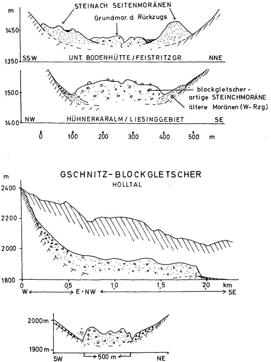
Abb. 7: Die beiden oberen Querprofile zeigen die normale Entwicklung von Steinach-Moränen. Im Falle Feistritzgraben kamen typische Seiten- und Endmoränen zur Ablagerung, im Liesinggebiet ist bereits zur Zeit des Steinachstadiums der Übergang zu blockgletscherartigen (Grund-) Moränenformen erkennbar; es fehlen jedoch die charakteristischen Wülste der Blockgletscher.
