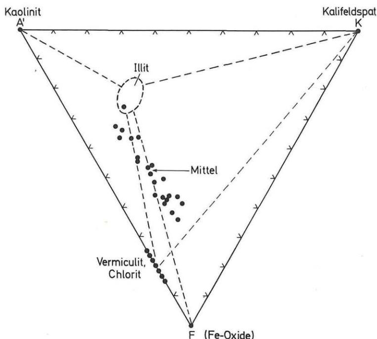
Abb. 6: In das A'KF-Dreieck nach Eskola sind wichtige Mineralien des Verwitterungszyklus eingetragen. Aus der Lage der Projektionspunkte von 22 chemischen Analysen von Schiefergneisen-Glimmerschiefen der Koralpe kann gesehen werden, daß diese Gesteine aus den beiden Hauptmineralien für Schiefertone, Illit und Chlorit, GRIM 1968:554, mit Einstreuungen von Kalifeldspat und Kaolinit \pm Erzen dargestellt werden können. Einstreuungen von Quarz und Plagioklas sind durch das verwendete Diagramm nicht erfäßbar.
