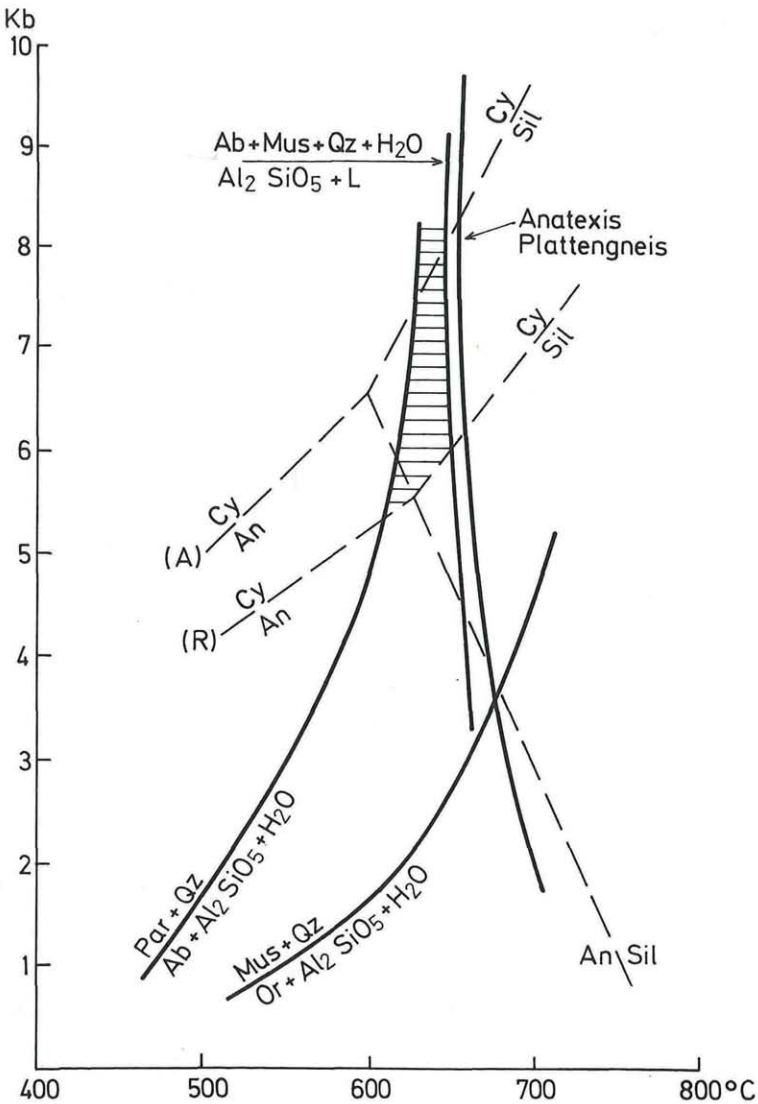
Abb. 5: Gleichgewichtsbedingungen einiger für die Metamorphose von Schiefergneisen-Glimmerschiefern der Koralpe wichtiger Reaktionen. \text{Al}_2\text{SiO}_5 -Modifikationen nach ALTHAUS 1967, 1969a, 1969b (A) und nach RICHARDSON et al. 1968, 1969 (R); Paragonit + Quarz = Albit + \text{Al}_2\text{SiO}_5 + \text{H}_2\text{O} nach CHATTERJEE 1972; Muskowit + Quarz = Kalifeldspat + \text{Al}_2\text{SiO}_5 + \text{H}_2\text{O} nach ALTHAUS et al. 1970; Albit + Muskowit + Quarz + \text{H}_2\text{O} = \text{Al}_2\text{SiO}_5 + Schmelze nach STORRE & KAROTKE 1971; Anatexis des Plattengneises nach PLATEN & HÜLLER 1966. Der schraffierte Bereich entspricht den wahrscheinlichen Bildungsbedingungen der Paragenese Cyanit + Albit + Quarz + Muskowit, die in der Koralpe in Schiefen mit Cyanitparamorphosen nach Andalusit beobachtet werden kann.
