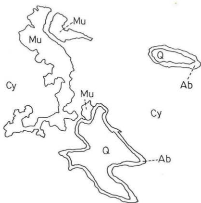
Abb. 4: In einer Paramorphose von Cyanit (Cy) nach Andalusit wird Muskowit (Mu) neben Quarz (Q) und Albit (Ab) beobachtet. Reaktionssäume um Quarz lassen eine Reaktion Cyanit und Quarz zu Albit erkennen, wobei, offenbar an Intergranularen, Na-Ion hinzu diffundiert; 4a gekreuzt polarisiertes Licht, 4b Zuordnung der Mineralien.
