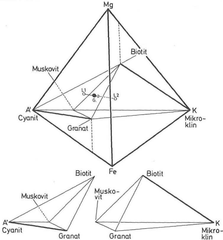
Abb. 2: Erweiterung des A'KF-Dreiecks nach Eskola zum A'KF Fe Mg-Tetraeder. Die Projektionspunkte von Granat und Biotit liegen in den entsprechenden Ebenen des Tetraeders und weisen etwa die von PACHER & RIEPL 1978 gefundene Zusammensetzung aus. Die 22 chemischen Analysen von Schiefergneisen-Glimmerschiefern der Koralpe liegen innerhalb der beiden Ebenen: Cyanit-Mikroklin-Biotit und Cyanit-Mikroklin-Granat. Zusammensetzungen links der entscheidenden Ebene Granat-Biotit-Muskowit haben den Mineralbestand L1 mit Muskowit + Biotit + Granat + Cyanit, Zusammensetzungen rechts der Ebene Granat-Biotit-Muskowit haben den Mineralbestand L2 mit Mikroklin + Muskowit + Biotit + Granat; der Gehalt an Quarz und Plagioklas ist in der Darstellung nicht erfassbar. Feinlagige Gneise haben eine Gesamtzusammensetzung G, die meist knapp über der Ebene Granat-Biotit-Muskowit liegt; diese Gesamtzusammensetzung tritt in die Lagen L1 und L2 auseinander. Zur Verdeutlichung ist der Tetraeder-Raum Cyanit-Granat-Mikroklin-Biotit auch gesprengt dargestellt.
