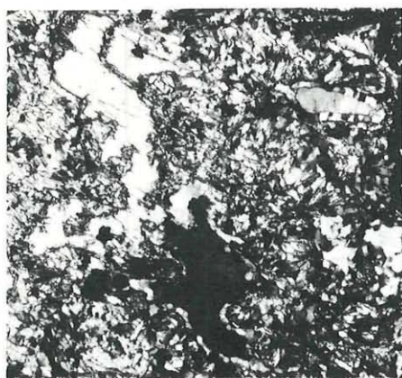
Abb. 4: In einer Paramorphose von Cyanit (Cy) nach Andalusit wird Muskowit (Mu) neben Quarz (Q) und Albit (Ab) beobachtet. Reaktionssäume um Quarz lassen eine Reaktion Cyanit und Quarz zu Albit erkennen, wobei, offenbar an Intergranularen, Na-Ion hinzu diffundiert; 4a gekreuzt polarisiertes Licht, 4b Zuordnung der Mineralien.
