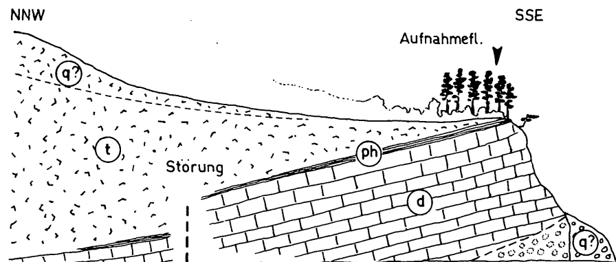
Abb. 2: Vereinfachtes geologisches Profil vom Südfuß des Annaberges bei Leoben (Zeichenerklärung im Text).
