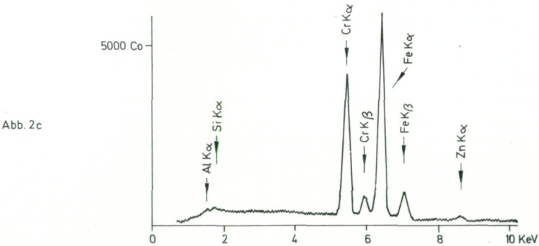
Abb. 2b und Abb. 2c: Elektronenstrahlmikroanalysen an den in Abb. 2a angegebenen Stellen. An diesem Korn ist fast keine Zonarität festzustellen. Die hauptsächlichsten Elemente Cr und Fe gestatten es, einen Mischkristall mit 0,48 Chromit und 0,52 Magnetit zu berechnen, wobei die sehr geringen Anteile von Zn bzw. Al und Si unberücksichtigt bleiben.
