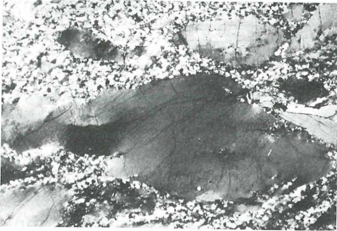
Abb. 1: Die lichtoptische Aufnahme zeigt Alkalifeldspat aus dem Plattengneis des Steinbruches Pretner. Eine mechanische Beanspruchung bewirkt einmal die Zerbrechung eines ursprünglich noch größeren Feldspates in die großen, undulös auslöschenden Körner und erzeugt weiterhin ein feinkörniges, rekristallisiertes Alkalifeldspat-Zerreibsel zwischen den großen Körnern (Mörtelkränze). Die Entmischungslamellen in den großen Körnern sind bei der gegebenen Vergrößerung nicht erkennbar. Der untere Rand der Abbildung ist in der Natur 6,5 mm lang.
