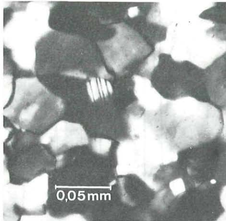
Abb. 8: Aus einem Mörtelkranz: Lichtmikroskopische Aufnahme, gekreuzt polarisiertes Licht, eines Albitkornes mit polysynthetischer Albitverzwillingung in einem kristalloblastischen Gefüge von vorwiegend Alkalifeldspat.
