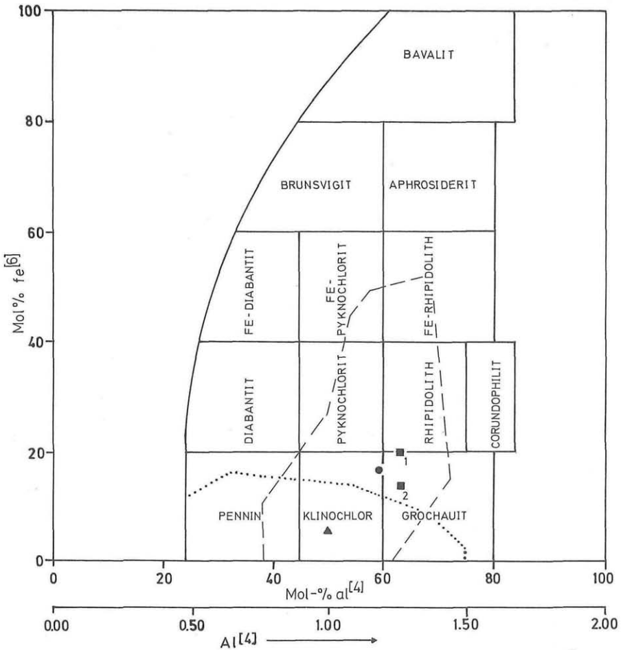
Abb. 1: Chemisches Variationsdiagramm der Orthochlorite (14 Å-Chlorite oder Normal-Chlorite mit niedrigen Eisen-(III)-Gehalten) und chemische Variation der Normal-Chlorite in Gesteinsvorkommen der magmatischen Abfolge (Chlorite in Serpentiniten und Peridotiten) bzw. der metamorphen Abfolge (Chlorite in Grünschiefern, Chloritschiefern und Amphiboliten) nach TRÖGER & TROCHIM 1967. Eingetragen ist der Chlorit vom Ochsenkogel aus der Gleinalpe (chemisch- und röntgenographisch bestimmt) und der Klinochlor aus Serpentiniten des Gleinalpengebietes nach ANGEL 1924.
