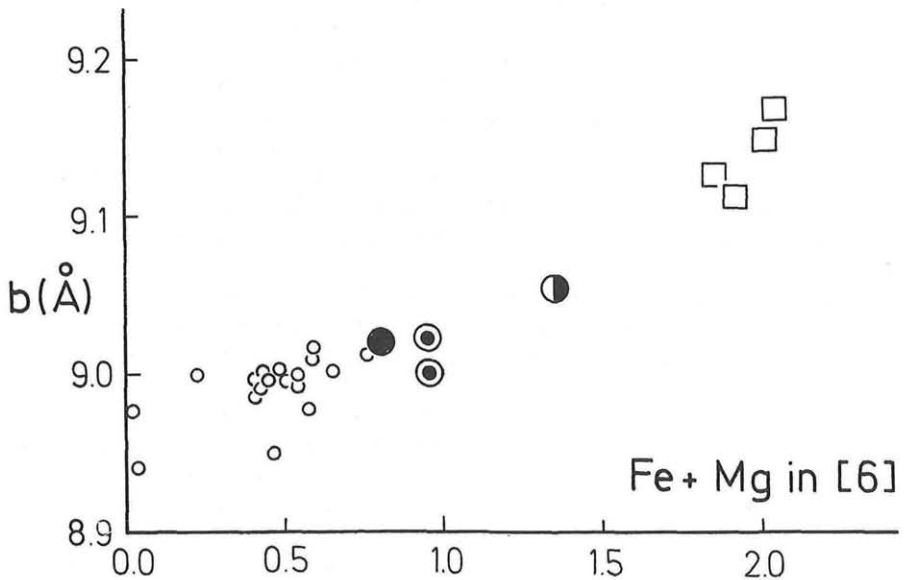
Abb. 2: Nach AOKI et al. 1974 ist die Gitterkonstante b (Å) gegen gesamt \text{Fe} + \text{Mg} eingetragen. Auch hier fügt sich der Ferrimontmorillonit aus der Gleichenberger Klause dem Trend von Montmorillonit zu Nontronit ein. Symbole wie in Abb. 1.
