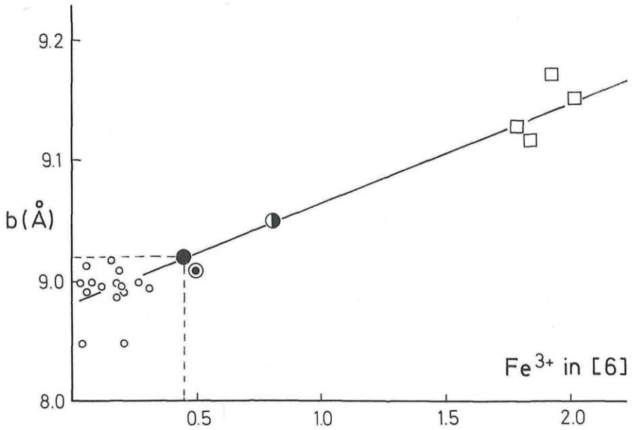
Abb. 1: Abhängigkeit der Gitterkonstante b (Å) von \text{Fe}^{3+} in [6]-Koordinat in dioktaedrischen Smectiten nach AOKI et al. 1974. Für den Ferrimontmorillonit aus der Gleichenberger Klause (Symbol: ausgefüllter Kreis) ist die o. a. Abhängigkeit sehr gut erfüllt. Weitere Symbole, leere Kreise: Montmorillonit-Beidellit, Kreise mit Mittelpunkt: eisenreicher Montmorillonit, halbgefüllter Kreis: Fe-Montmorillonit, Quadrate: Nontronit (AOKI et al. 1974).
