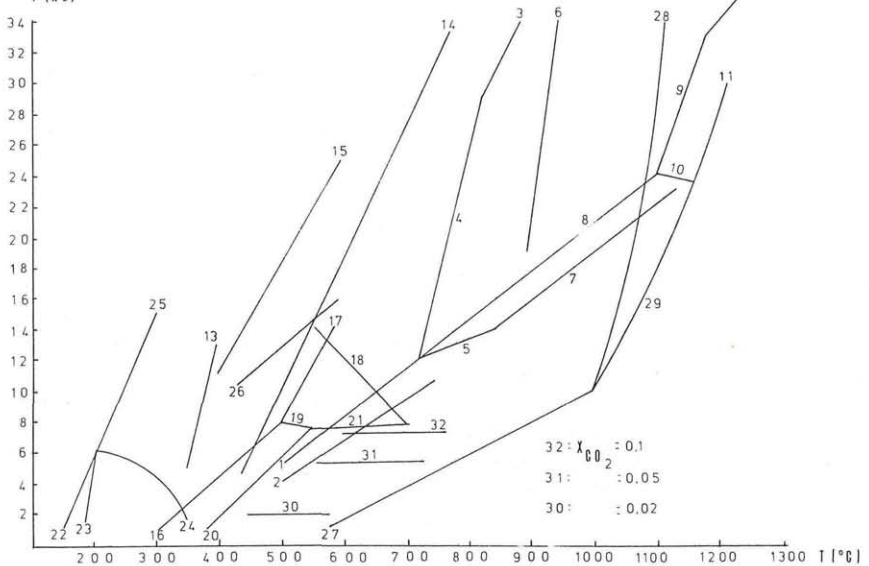
Abb. 1: Darstellung der Zoisit-Reaktion im Bereich von 150°C bis 1270°C und zwischen 1–34 kb. Die Reaktionen 1–12, 28, 29 nach BOETTCHER 1970, Nr. 16 bis 21 nach CHATTERJEE 1976, Nr. 15 nach HOLLAND 1979, Nr. 14 nach NEWTON & KENNEDY 1963, Nr. 13 nach NITSCH 1968, Nr. 22–27 nach PERKINS & WESTRUM & ESSENE 1980, Nr. 30–32 nach STORRE & NITSCH 1972.
