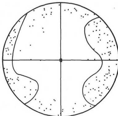
D 2: 149 Kalzitfugen, Koralm-Marmor senkrecht B.
