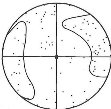
D 1: 100 Kalzitachsen, Koralm-Marmor senkrecht B.
