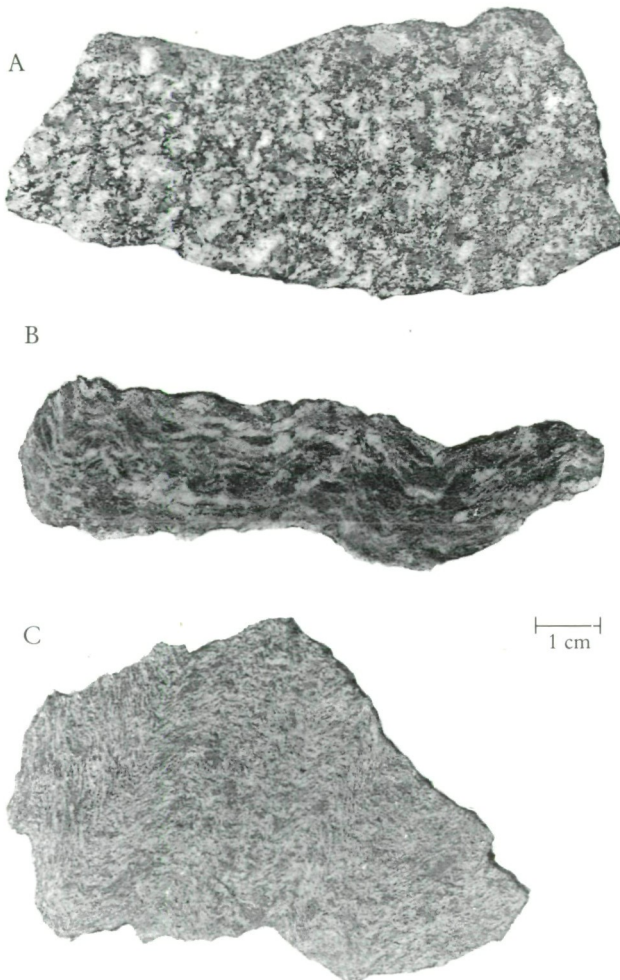
Abb. 1: „Metablastische“ Amphibolit-Typen A, B und C aus dem Kristallin der Gleinalpe, Rachau-graben.
