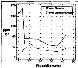
Abb. 13 a, b, c: Cr-, Mn- und Zn-Gehalt der unmagnetischen und der Gesamtfraction entlang der Murz
