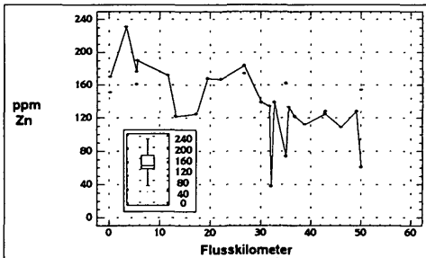
Abb. 11: Zn-Gehalte der Mürz; Längsprofil und Box-Plot
