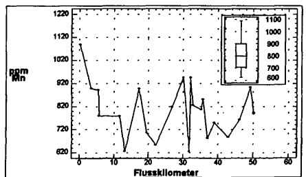
Abb. 8: Mn-Gehalt der Mürz; Längsprofil und Box-Plot
