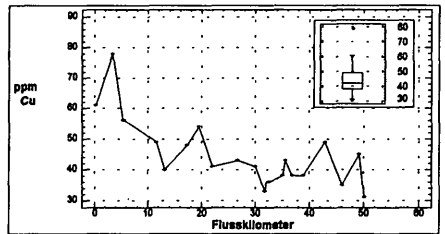
Abb. 6: Cu-Gehalte der Mürz; Längsprofil und Box-Plot
