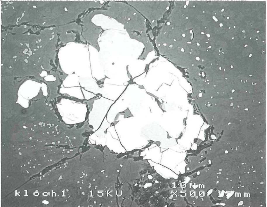
Abb. 9: Ilmenit mit gedrunzenen Rutilkristallen in Cordierit/Sekaniait mit Hercynit im Glas; Steinbruch Klöcher, Nördlicher Bruch, Klöcher Klause, Steiermark. REM-Foto: BSE-Bild. Bildbreite: 0,2 mm. Ilmenite with compact crystals of rutile in cordierite/sekaninaite with hercynite in a glassy matrix; Basaltquarry Klöcher, northern quarry, Klöcher Klause, Styria. BSE-image. Image width: 0,2 mm.
