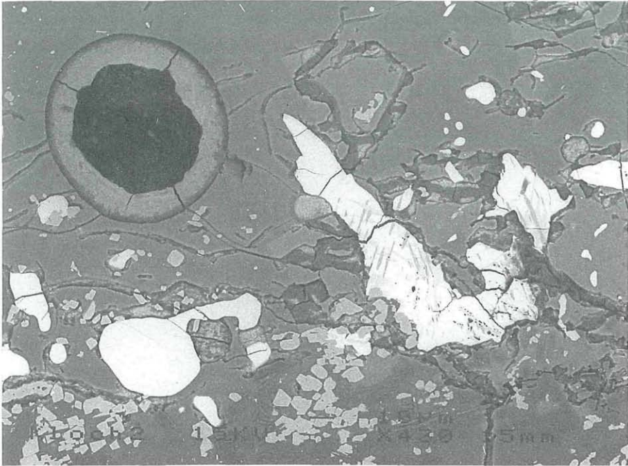
Abb. 10: Armalcolit (gerundet, links unten) mit Ilmenit, Rutil, Cordierit/Sekaninait, Hercynit sowie ein Tonmineral im Blasenraum im Glas; Steinbruch Klöch, Nördlicher Bruch, Klöcher Klause, Steiermark. REM-Foto: BSE-Bild. Bildbreite: 0,08 mm.
