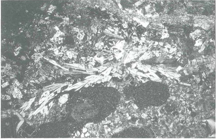
Abb. 2: Sanidin mit Cordierit/Sekaniait, Hercynit und Nontronit im Glas; Steinbruch Klöch, Nördlicher Bruch, Klöcher Klause, Steiermark. + Polarisatoren. Bildbreite: 2,5 mm. Sanidine with cordierite/sekaninaite, hercynite and nontronite in glass; Basaltquarry Klöch, northern quarry, Klöcher Klause, Styria. Crossed polars. Image width: 2,5 mm.
