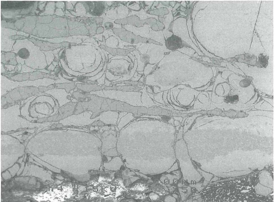
Abb. 1: Glas mit perlitischer Struktur mit Al-reichen Mineralphasen (schmale graue Lagen) sowie Quarz; Steinbruch Klöch, Nördlicher Bruch, Klöcher Klause, Steiermark. REM-Foto: BSE-Bild. Bildbreite: 1 mm.
