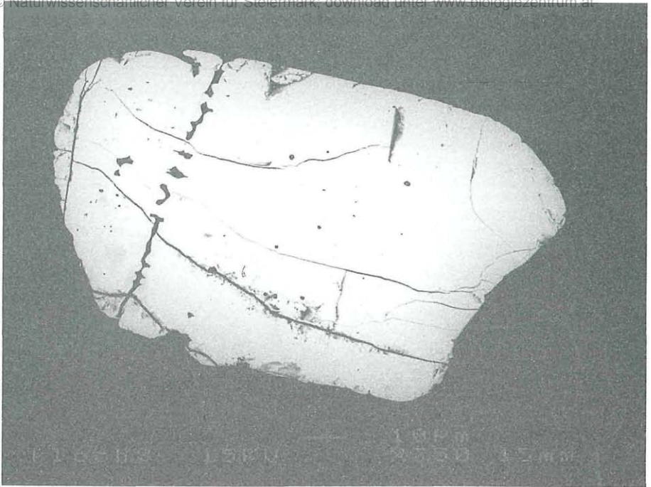
Abb. 13: Chemisch inhomogener Monazit-(Ce) (Cheralith) im Glas; Steinbruch Klöch, Nördlicher Bruch, Klöcher Klause, Steiermark. REM-Foto: BSE-Bild. Bildbreite: 0,2 mm. Chemical inhomogeneous monazite-(Ce) (cheralite) in glass; Basaltquarry Klöch, northern quarry, Klöcher Klause, Styria. BSE-image. Image width: 0,2 mm.
