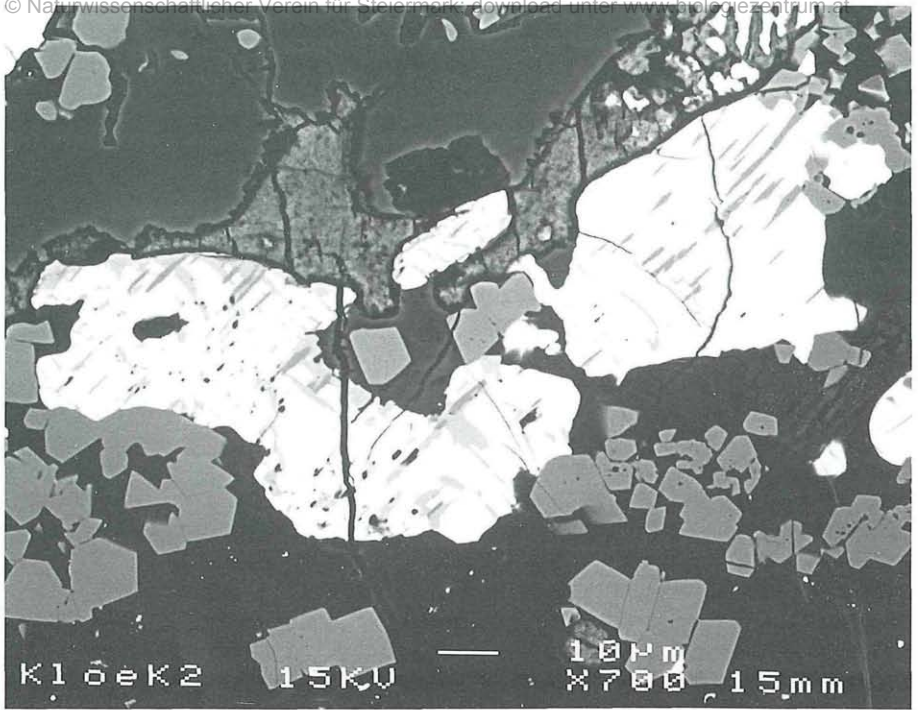
Abb. 16: Orientiert eingelagerter Rutil im Ilmenit mit Hercynit und Monazit-(Ce) (Cheralith) und Tonmineral im Glas; Steinbruch Klöch, Nördlicher Bruch, Klöcher Klause, Steiermark. REM-Foto: BSE-Bild. Bildbreite: 0,14 mm. Oriented intergrowth of rutile with ilmenite as well as hercynite, monazite-(Ce) (cheralite) and a clay mineral in glass; Basaltquarry Klöch, northern quarry, Klöcher Klause, Styria. BSE-image. Image width: 0,14 mm.
