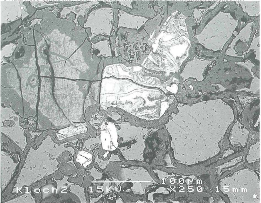
Abb. 18: Relikte des Ti-reichsten Magnetits mit Zonierung von Ti-reichem Glas? umgeben mit Ilmenit und Halloysitkrusten im Glas; Steinbruch Klöch, Nördlicher Bruch, Klöcher Klause, Steiermark. REM- Foto: BSE-Bild. Bildbreite: 0,5 mm.
