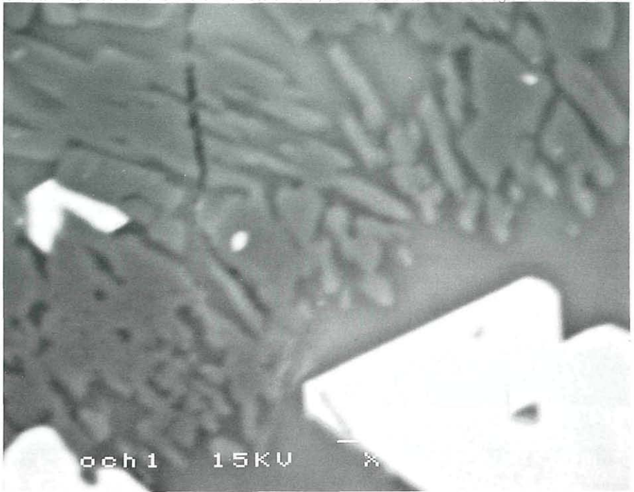
Abb. 3: Blockige und stäbchenartige Kristalle und Aggregate von \text{Al}_2\text{SiO}_5 -Mineralphasen mit Hercynit im Glas; Steinbruch Klöch, Nördlicher Bruch, Klöcher Klause, Steiermark. REM-Foto: BSE-Bild. Bildbreite: 0,003 mm.
