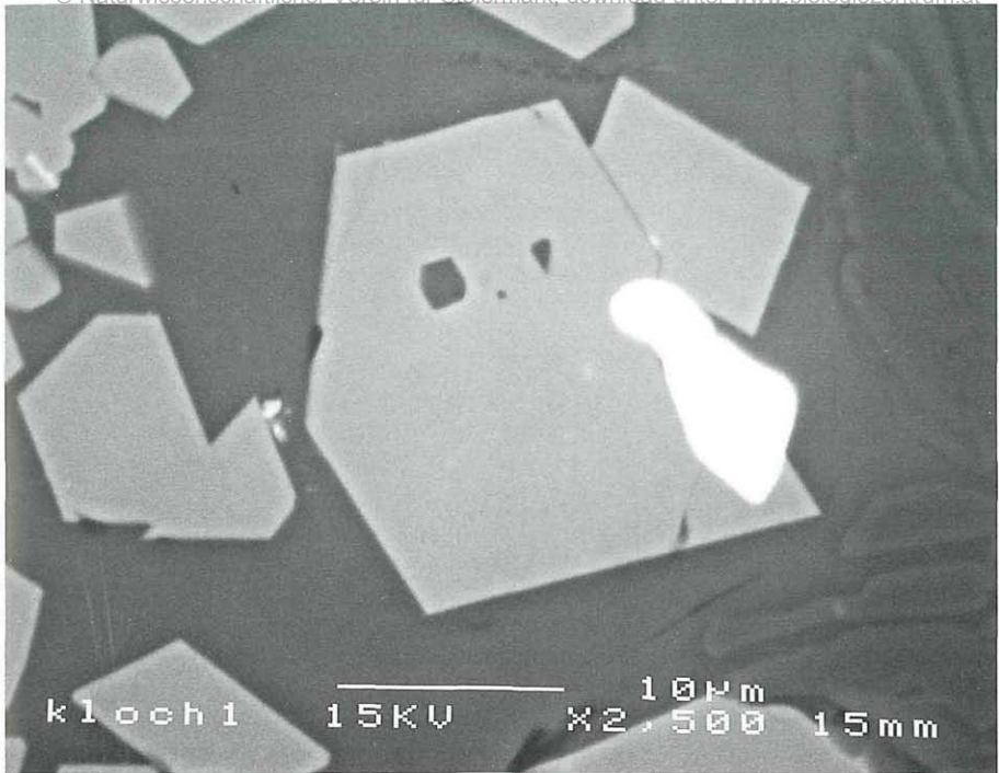
Abb. 8: Hercynitkristall mit Zirkon im Glas; Steinbruch Klöch, Nördlicher Bruch, Klöcher Klausen, Steiermark. REM-Foto: BSE-Bild. Bildbreite: 0,05 mm. Hercynite with zircon in a glassy matrix; Basaltquarry Klöch, northern quarry, Klöcher Klausen, Styria. BSE-image. Image width: 0,05 mm.
