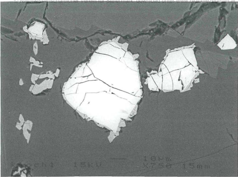
Abb. 12: Ilmenit mit Ferrosilit umwachsen gemeinsam mit Cordierit/Sekaninaït im Glas; Steinbruch Klöch, Nördlicher Bruch, Klöcher Klaus, Steiermark. REM-Foto: BSE-Bild. Bildbreite: 0,2 mm. Ferrosilite grows around ilmenite with cordierite/sekaninaite in glass; Basaltquarry Klöch, northern quarry, Klöcher Klaus, Styria. BSE-image. Image width: 0,2 mm.
