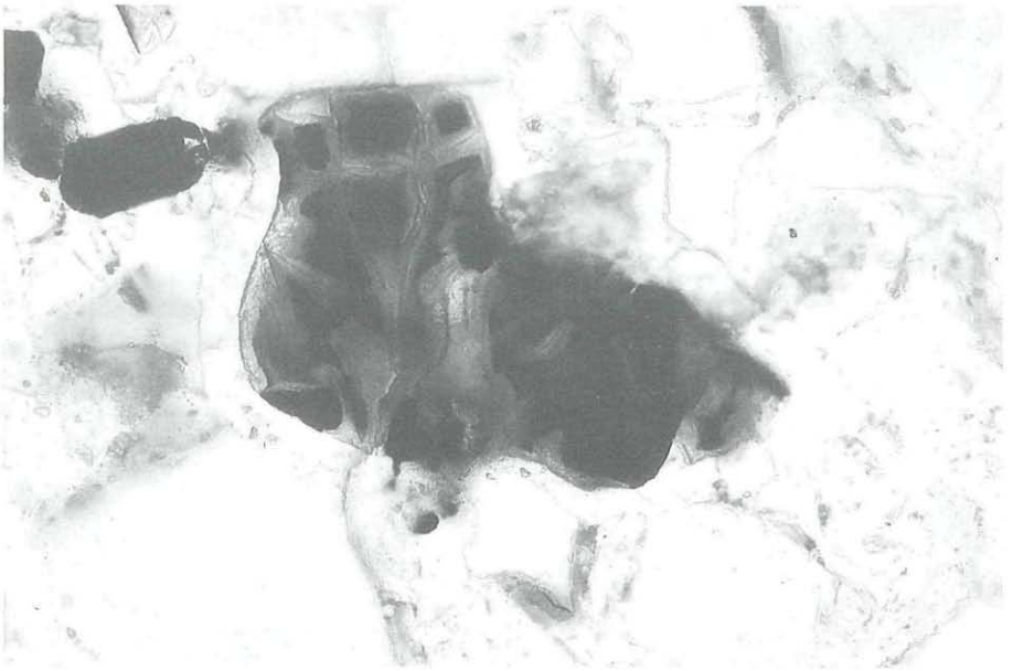
Abb. 19: Ti-reiches Glas? um extrem Ti-hältigen Magnetit; Steinbruch Klöch, Nördlicher Bruch, Klöcher Klause, Steiermark. Bildbreite: 0,32 mm. Ti-rich glass rimming high-grade Ti-magnetite; Basaltquarry Klöch, northern quarry, Klöcher Klause, Styria. BSE-image. Image width: 0,32 mm.
