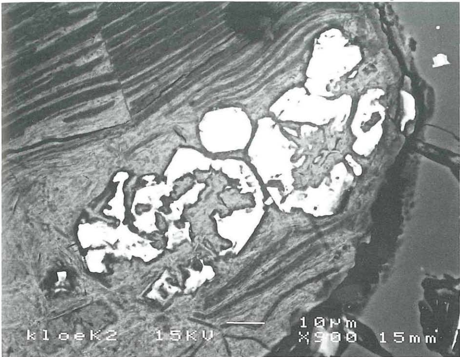
Abb. 17: Reliktischer Magnetit mit Pyrit im Nontronit einer Blasenfüllung im Glas; Steinbruch Klöch, Nördlicher Bruch, Klöcher Klause, Steiermark. REM-Foto: BSE-Bild. Bildbreite: 0,12 mm. Relict magnetite with pyrite in nontronite in a glass cavity; Basaltquarry Klöch, northern quarry, Klöcher Klause, Styria. BSE-image. Image width: 0,12 mm.
