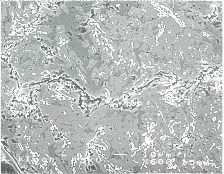
Abb. 5: Hercynit myrmekitartig mit Cordierit/Sekaninait verwachsen im Glas; Steinbruch Klöch, Nördlicher Bruch, Klöcher Klause, Steiermark. REM-Foto: BSE-Bild. Bildbreite: 0,2 mm. Myrmecitic intergrowth of hercynite with cordierite/sekaninaite in glass; Basaltquarry Klöch, northern quarry, Klöcher Klause, Styria. BSE-image. Image width: 0,2 mm.
