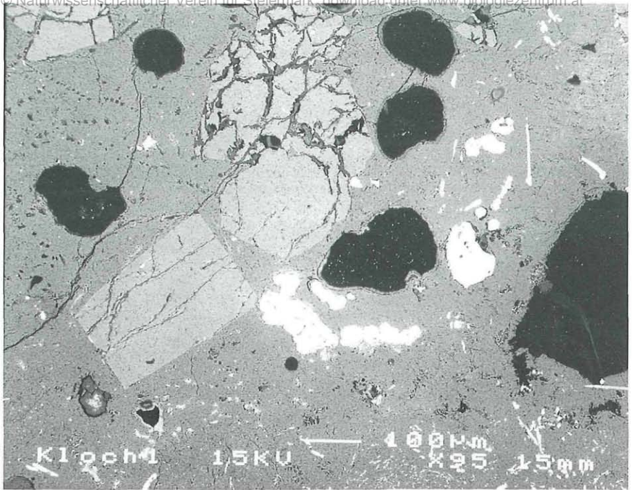
Abb. 7: Cordierit/Sekaninaitkristalle (C2) mit Ilmenit im Glas; Steinbruch Klöch, Nördlicher Bruch, Klöcher Klause, Steiermark. REM-Foto: BSE-Bild. Bildbreite: 1,1 mm. Crystals of cordierite/sekaninaite (C2) with ilmenite in glass; Basaltquarry Klöch, northern quarry, Klöcher Klause, Styria. BSE-image. Image width: 1,1 mm.
