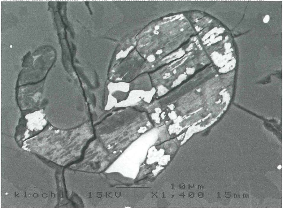
Abb. 11: Magnetit mit Ilmenit und Monazit-(Ce) (Cheralith) im Nontronit in einem Blasenhohlraum im Glas; Steinbruch Klöch, Nördlicher Bruch, Klöcher Klaus, Steiermark. REM-Foto: BSE-Bild. Bildbreite: 0,3 mm.
