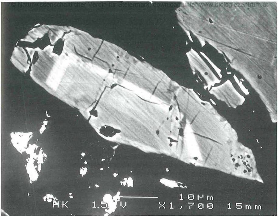
Abb. 6: Xenotim mit oszillierendem Zonarbau. Probe HK1fa, BSE-Bild, Bildbreite 0,07 mm. Oscillatory zoned xenotime, sample HK1fa, BSE image, width of photo 0,07 mm.
