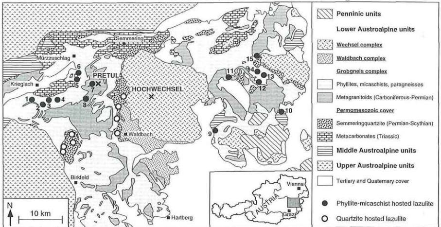
Abb. 1: Vereinfachte geologische Karte des unterostalpinen Deckenstapels in Ostösterreich nach NEUBAUER & al. 1992 mit den wichtigsten Lazulithvorkommen. 1 Freßnitzkogel, 2 Rotriegel, 3 Freßnitzgraben, 4 Höllkogel, 5 Fürstenbauer, 6 Ganztal, 7 Amundsenhöhe, 8 Grossmarker, 9 Schäffern, 10 Kirchschiach, 11 Krumbach, 12 Thal, 13 Spratzau A, 14 Spratzau B, 15 Stickelberg (aus BERNHARD & al. 1998).
