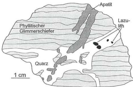
Abb. 4: Eine schmale, lazulithführende Quarzader durchschlägt diskordant ihr Nebengestein, daneben ist ein jüngeres Apatitmobilisat zu erkennen. Skizze nach angeschliffenem Handstück, Probe FG18, Freßnitzgraben.
