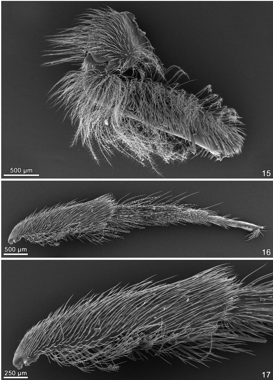
Abb. 15–17: Colletes hederiae , Weibchen, linkes Hinterbein. – Abb. 15. Blick auf die Außenseite (Vorderseite) schräg von unten mit Coxa, Trochanter und Femur, entlang der sichtbaren Kante des Femur liegt die kahle Fläche der Corbicula. – Abb. 16. Vorderseite von Tibia und Tarsus. – Abb. 17. Detail aus Abb. 16, Scopa auf Tibia und Metatarsus (nur Basis sichtbar). – Fotos: E. STABENTHEINER.
