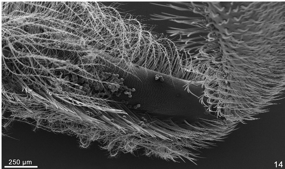
Abb. 13–14: Colletes hederae , Weibchen, rechtes Hinterbein ungefähr von unten mit Blick in die Corbicula. – Abb. 13. Von links nach rechts: Coxa, Trochanter und Femur; rechts außen Tibia und Metatarsus, die schräg stehen und daher optisch verkürzt erscheinen. – Abb. 14. Detail aus Abb. 13, femorale Corbicula und basaler Teil der Tibia mit Scopa. – Fotos: E. STABENTHEINER.
