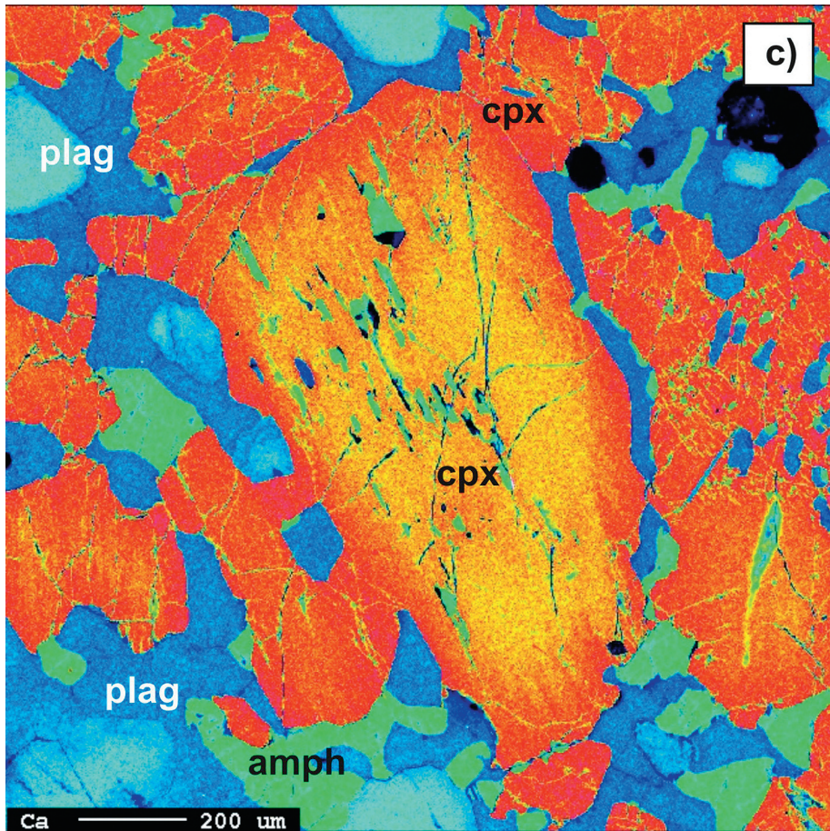
Abb. 2: c) Verteilung von Ca zwischen Klinopyroxen (cpx), Plagioklas (plag) und Amphibol (amph) in einem Granulit aus den Rhodopen. c) distribution map for Ca: clinopyroxene (cpx), plagioclase (plag) and amphibole (amph) in granulite from Rhodope.
