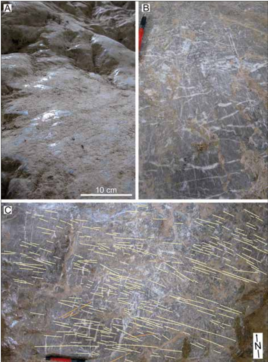
Abb. 2: Oberfläche des Dachsteinkalk-Untergrundes der Johanneskapelle nach Entfernung der Geschiebemergelaufage. (A) Spiegelglatt polierter Gletscherschliff. (B) Zahlreiche parallel verlaufende Gletscherschrammen auf der polierten Oberfläche dokumentieren die Bewegungsrichtung des Eises. (C) Es kommen zwei sich kreuzende Systeme von Gletscherschrammen vor (NW–SE, SW–NE). Schrammen mit NW–SE-Ausrichtung sind vorherrschend.
