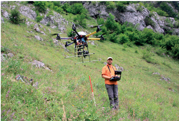
Abb. 3: E.C.O.pteryx im Einsatz. Der Hexakopter mit GPS-gestützter Flugsteuerung liefert hochauflösende Luftbilder von den Lebensräumen als Grundlage für die Geländekartierung. (Foto: E.C.O., Jungmeier)
