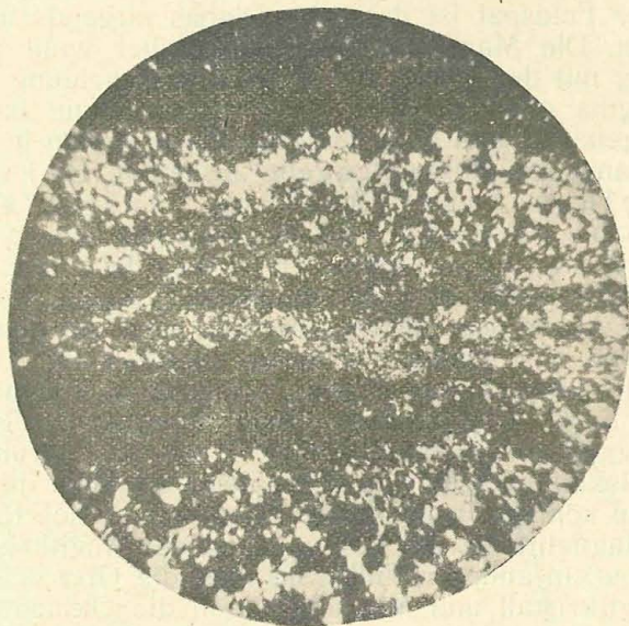
Abbildung 1: Magnetit-Feldspat-Verband in der liquidmagmatischen Magnetitlagerstätte der Platte bei Gatz 17 \times Vergr.
