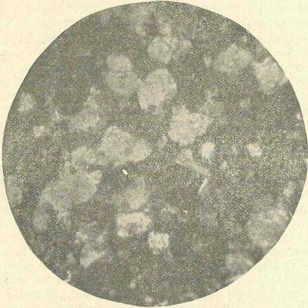
Abbildung 3: Liquidmagmatische Diabas - Magnetitlagerstätte vom Adam bei Mießdorf (Prevalje). Primäre Pyritwürfel aus der I. Ausscheidungsphase wurden von später gebildeten Chloritschuppen eingewickelt und teilweise in dieser Umrahmung verdreht und die dann entstandenen Zwickel mit neugebildetem Quarz ausgefüllt. Links unten ein Pyritwürfel, welcher von der einen Seite durch den später gebildeten Magnetit und von der anderen Seite durch Chlorit verdrängt wurde. Die Augite sind sämtlich chloritisiert. 17 × Vergr.
