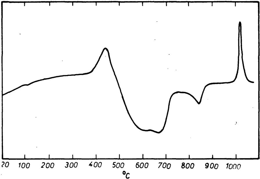
Abb. 2: D. T. A. - Kurve des nicht vorbehandelten Materials
