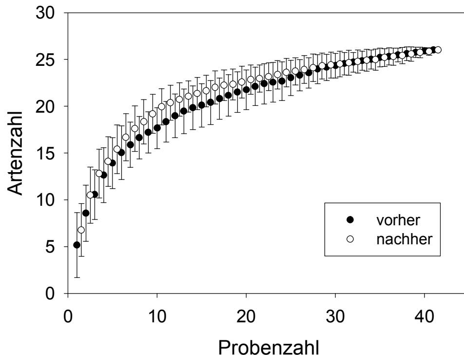
Abb. 3: Verlauf und Streuung (Mittelwert \pm Standardabweichung) der Artenzahl in Abhängigkeit von der Probenzahl.
