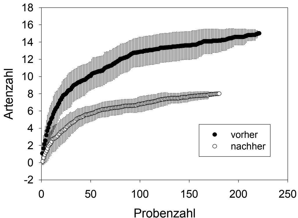
Abb. 8: Verlauf und Streuung (Mittelwert \pm Standardabweichung) der Artenzahl in Abhängigkeit von der Probenzahl.
