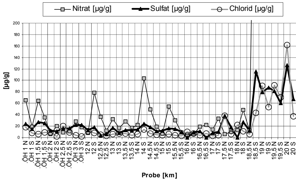
Abbildung 10: Verteilung von Nitrat, Sulfat und Chlorid im Längsverlauf des MFSD. Die Nitratwerte km 18-20 liegen oberhalb der gewählten Skala (600-700µg/g)
