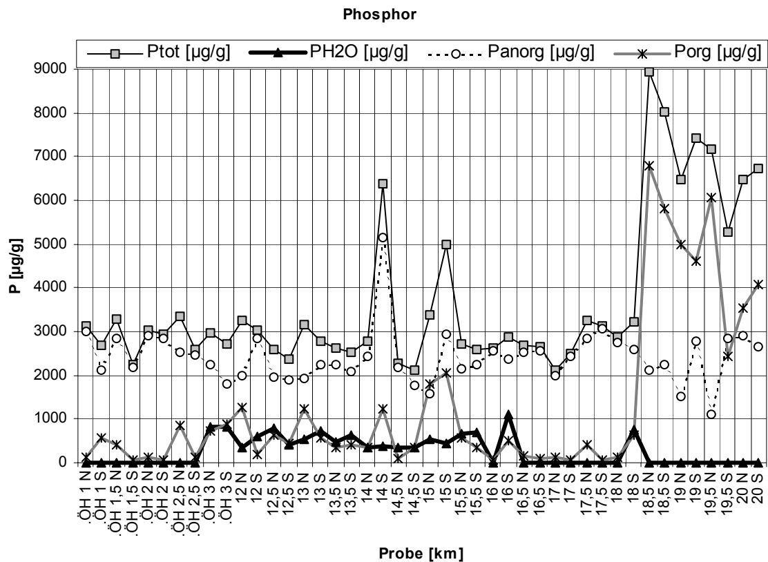
Abbildung 7: Verteilung der Phosphorfraktionen im Längsverlauf des MFSD.
