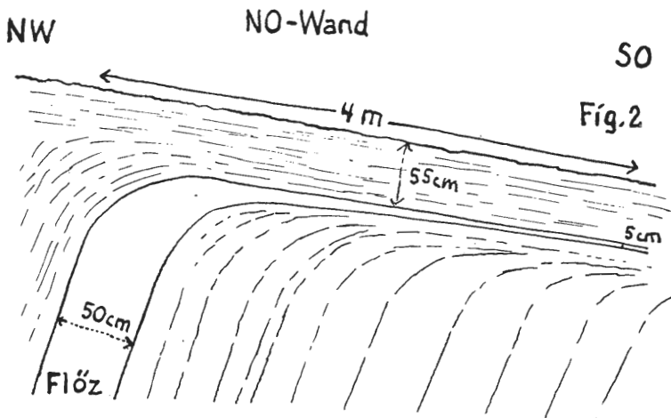
Fig. 2 Ausgehendes Kohlenflöz im Hangbodenfluß; es tritt auf der Erdoberfläche nicht in Erscheinung.
