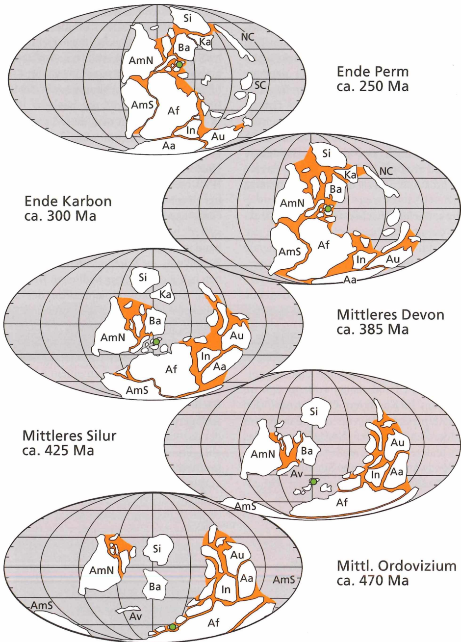
Abb. 3: Die Entstehung des Fundaments von Mitteleuropa im Paläozoikum. Grafiken modifiziert nach Darstellungen von SCOTESE ( www.scotese.com ), der Weg der Mikroplatten zum varistischen Gebirge nach FRANKE et al.2000. Festländische Kontinentalbereiche sind weiß bezeichnet. Die hellbraune Markierung verbindet kontinentale Bereiche, die als plattentektonische Einheit zusammengefasst werden können, wobei eine Bedeckung mit flachen Schelfmeeren möglich war. Abkürzungen: Aa/Antarktis, Af/Afrika, AmN/Nordamerika, AmS/Südamerika, Au/Australien, Av/Avalonia, Ba/Baltischer Schild, In/Indien, Ka/Kasachstan, NC/Nordchina, SC/Südchina, Si/Sibirischer Schild. Die Lage Nürnbergs (grüner Punkt) wäre am Rand oder zwischen zwei Mikroplatten („Saxothuringia“ und „Bohemia“ bzw. „Moldanubia“) anzusiedeln.
