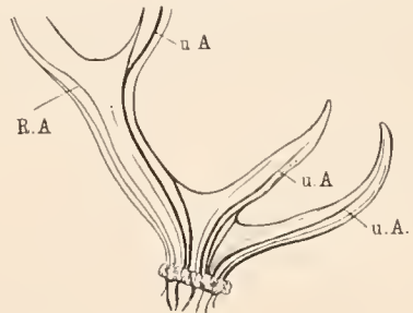
Fig. 5. Verlauf der Arterien auf dem unteren Teil einer rechtsseitigen Zelmenderstange (nach einem Injektionspräparat des Marburger zoologischen Instituts). RA = Arterien der Geweihrückenseite; uA = Arterien der unteren Konvexeiten der Sprossen.
