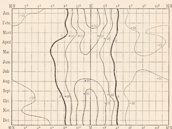
Fig. 2. Jährlicher Gang der Horizontalintensität in Samoa.
