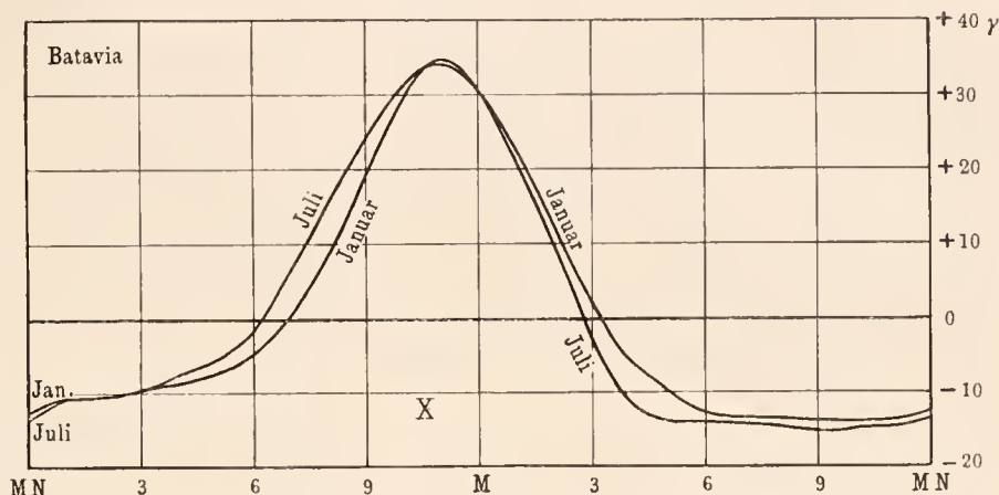
Fig. 6. Täglicher Gang der Nordkomponente in Batavia.
