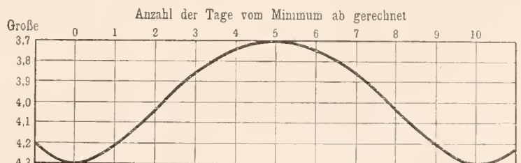
Fig. 4. Lichtkurve von \zeta Geminorum.
