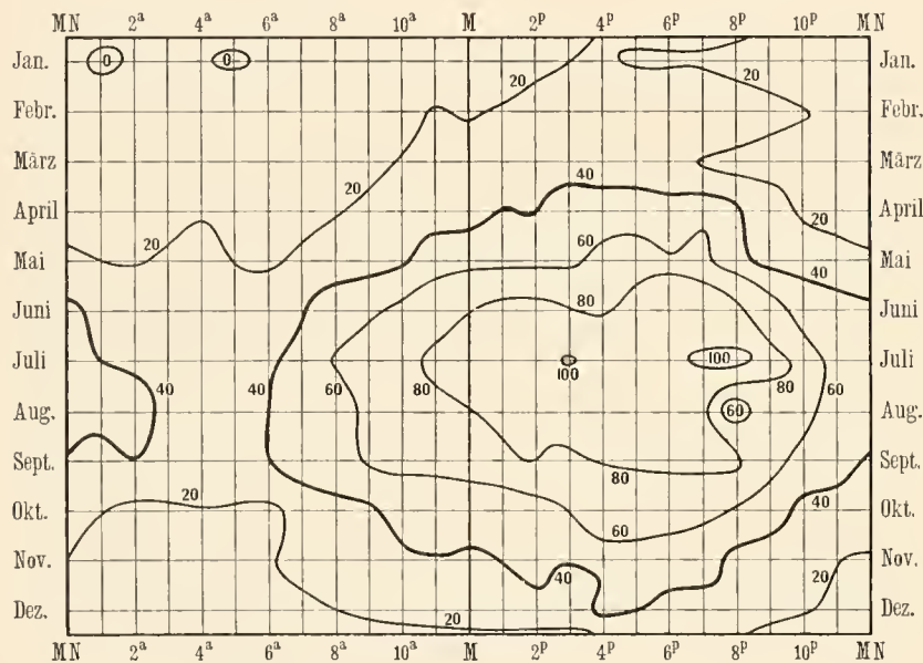
Täglicher und jährlicher Gang des lufterlektrischen Potentialgefälles in Samoa (1906 bis 1908) in Volt/m.
