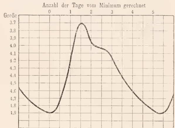
Fig. 3. Lichtkurve von \delta Cephei.
