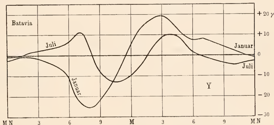
Fig. 7. Täglicher Gang der Westkomponente in Batavia.
