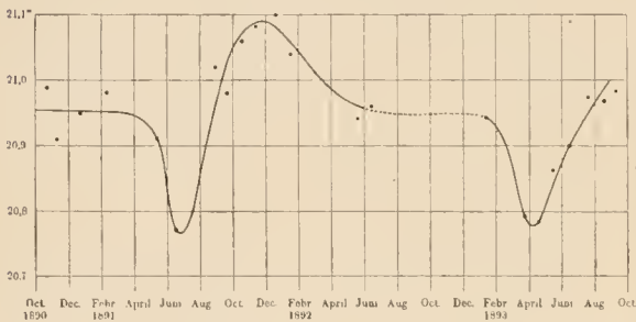
Veränderung des Abstandes der Componenten von 61 Cygni.
