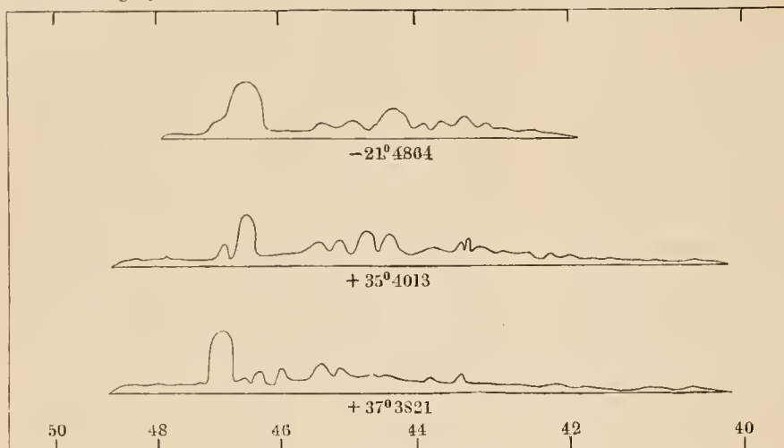
B. Photographische Intensitätscurven der Spectra einiger Wolf-Rayet-Sterne.
