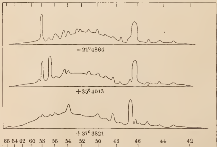
A. Optische Intensitätscurven der Spectra einiger Wolf-Rayet-Sterne.
