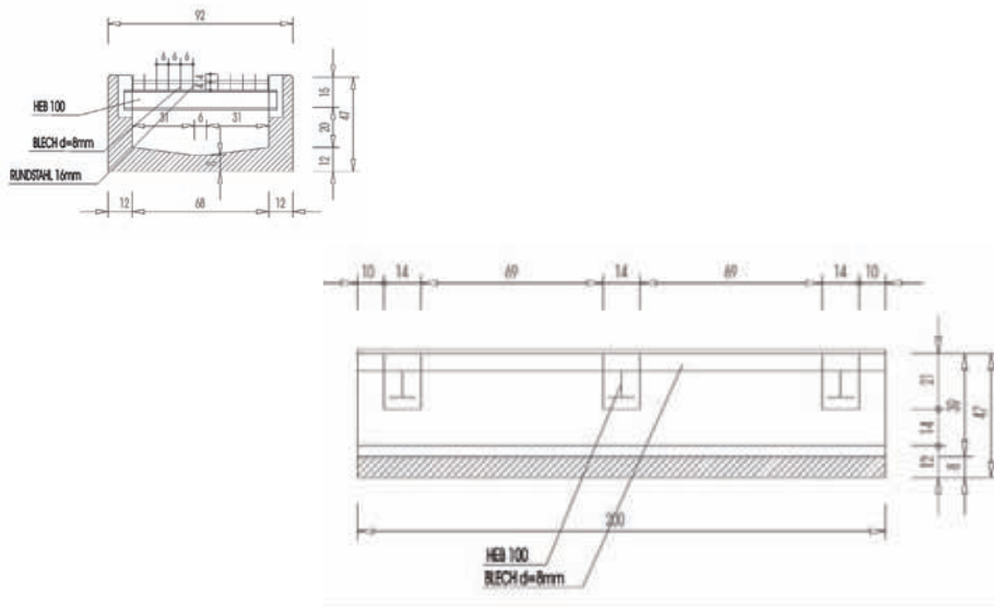
Abb. 7: Prinzipskizze und Maße eines Gitterrostes (SKIZZE: Büro FELBER-RICHTER, Salzburg)
