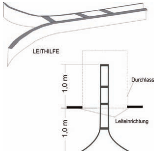
Abb. 10: Skizze zur Ausführung einer Leithilfe (Skizze: M. KYEK)
