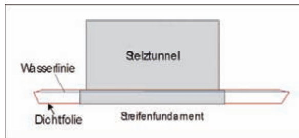
Abb. 5: Skizze zur Abdichtung eines Selztunnels (vgl. KYEK & WITTMANN 2004)
