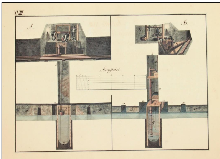
Abb. 13: Solehebung mit Pulgen und Handpumpe, Tafel XVIII aus M. Kefer 1836, Archiv Salinen Austria AG
